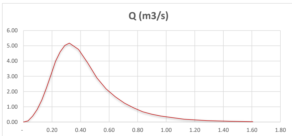
Gráfico 12. Hidrograma adimensional
