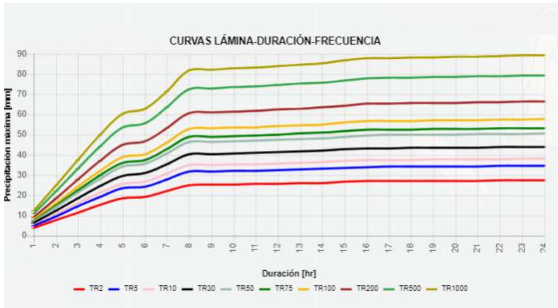
Gráfico 8. Curvas Lamina – Duración – Frecuencia ESCENARIO CAMBIO CLIMATICO RCP 8.5
