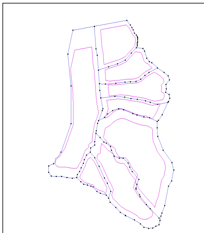
Figura 11: Generación de la superficie del modelo en Iber-2d
