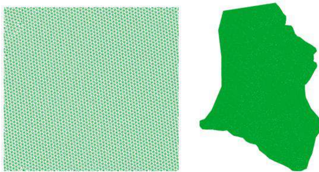
Figura 13 : Malla computacional del modelo hidráulico
