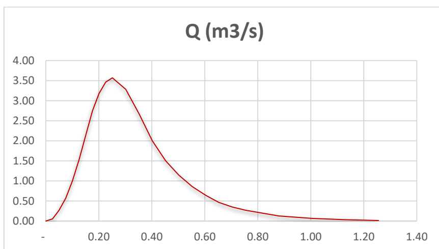
Gráfico 14. Hidrograma adimensional
