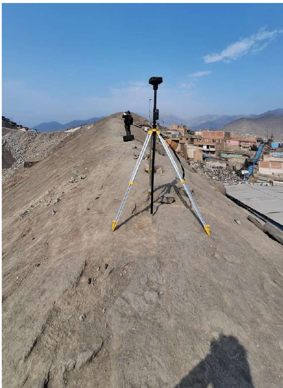
Figura 5. Levantamiento topográfico en el ámbito 3
