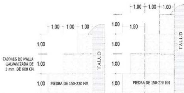
DETALLE MURO DE CONTENCION CON GAVIONES
