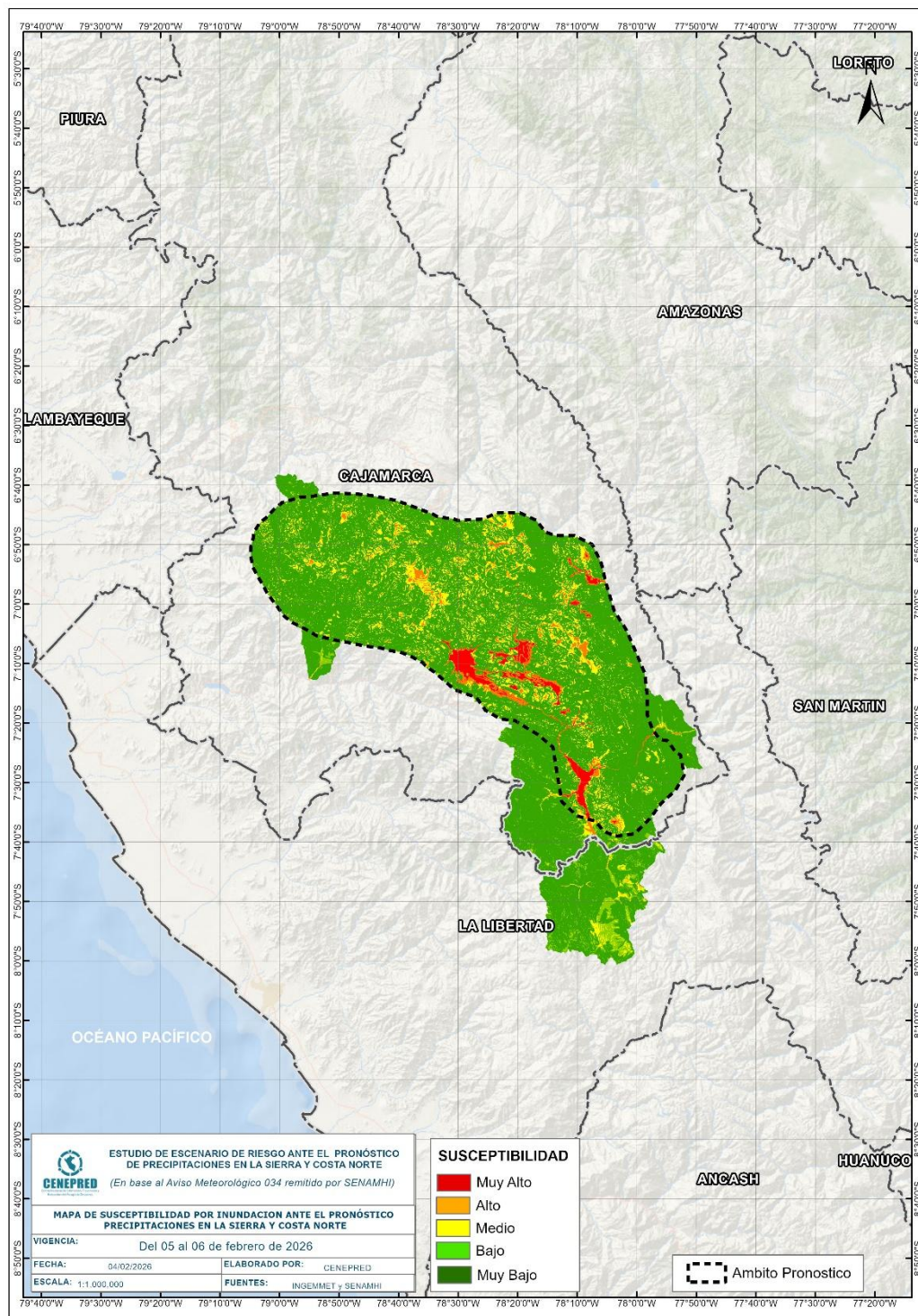
Figura 6. Escenario de riesgo por inundaciones en el ámbito del pronóstico de precipitaciones en la sierra y costa norte del 05 al 06 de febrero del 2026
