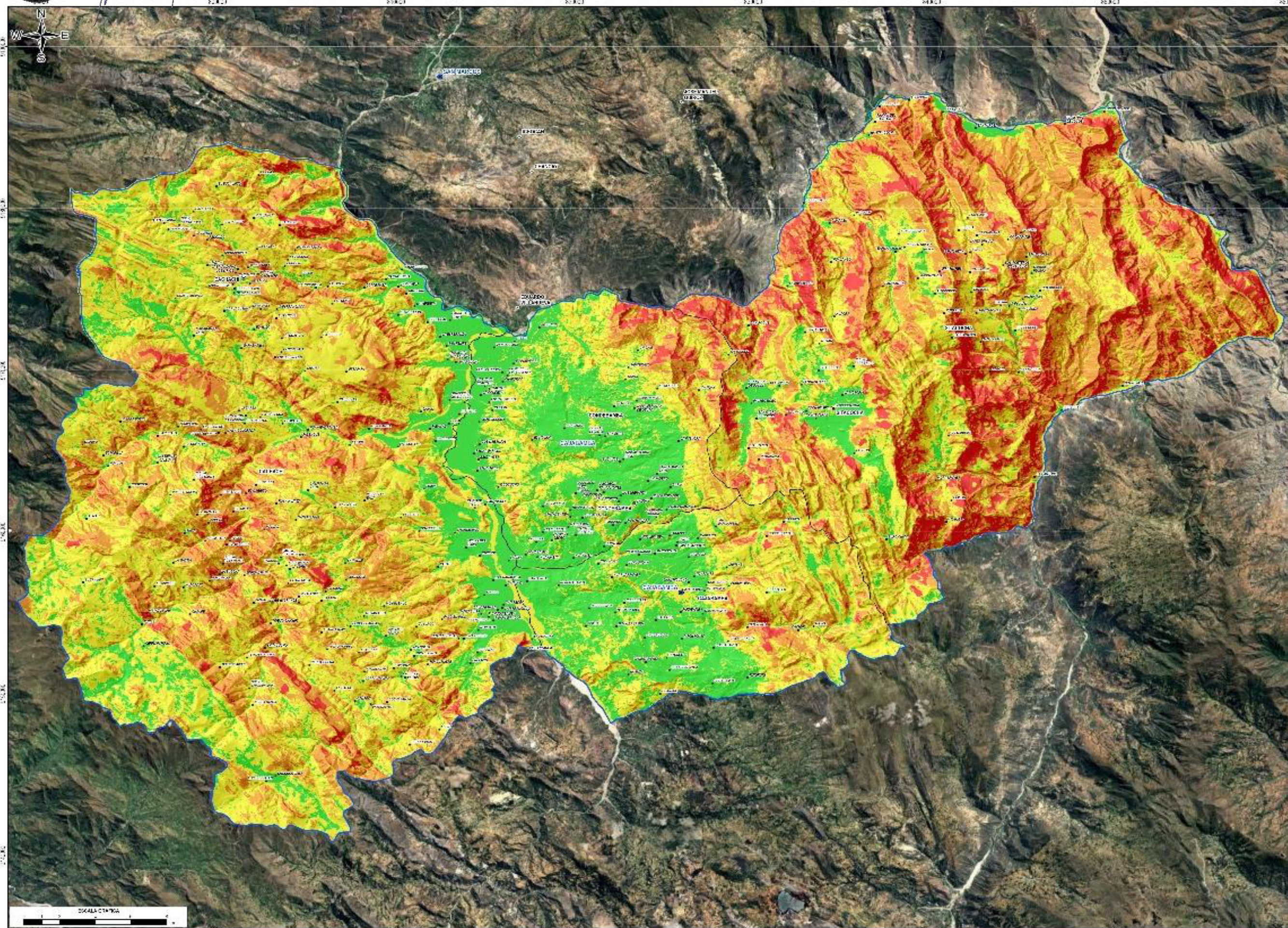
Mapa 15. Niveles de peligro – Deslizamiento
