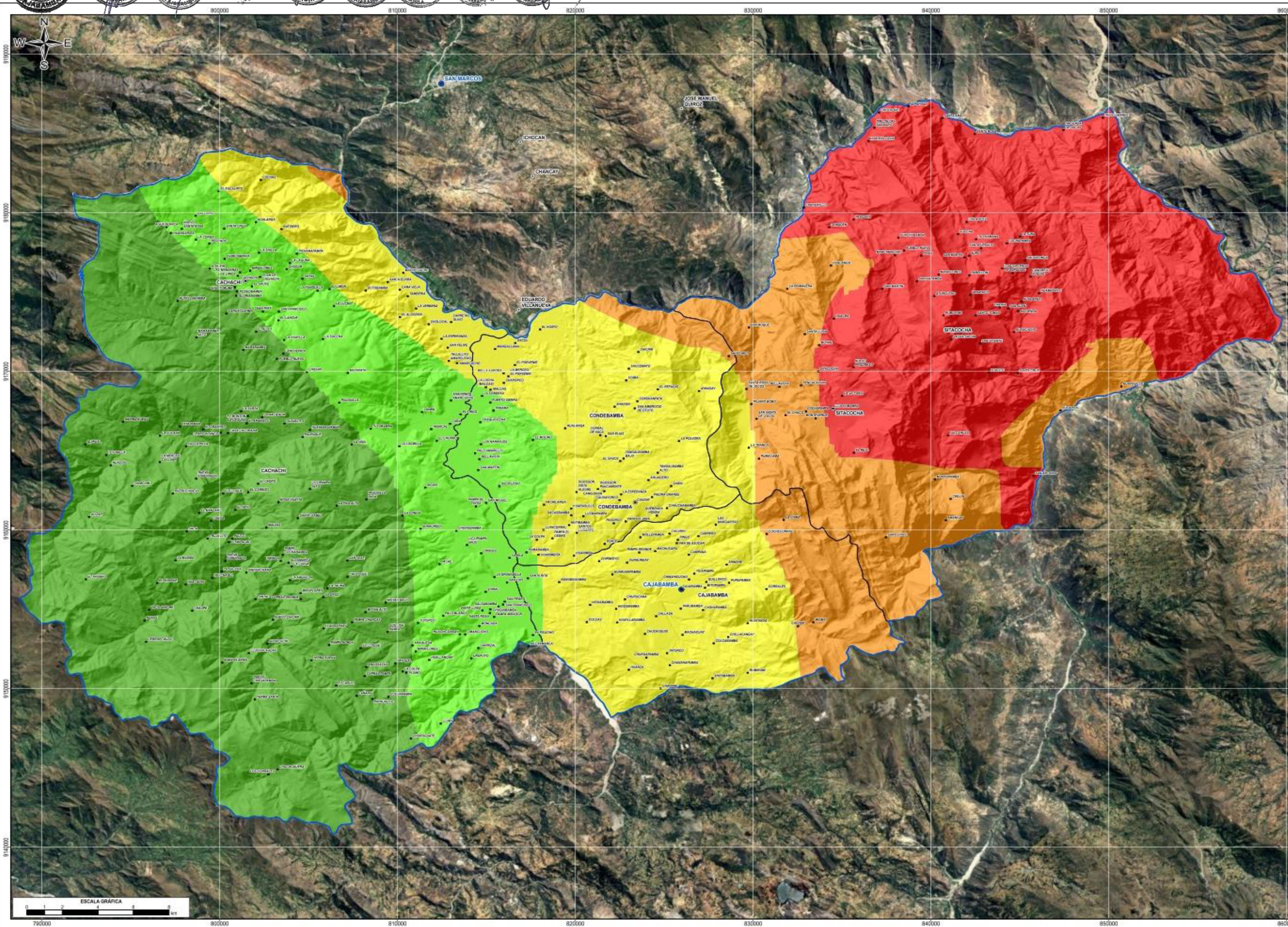
Mapa 12. Anomalías de precipitaciones FEN.
