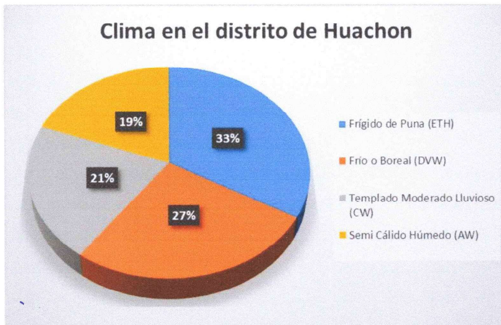
Figura 7. Distribución de Climas en el Distrito de Huachón
