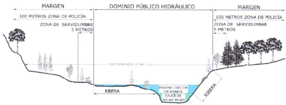
Figura 14. Sección típica simplificada de un río en la que se observa el canal principal, así como las llanuras de inundación.
