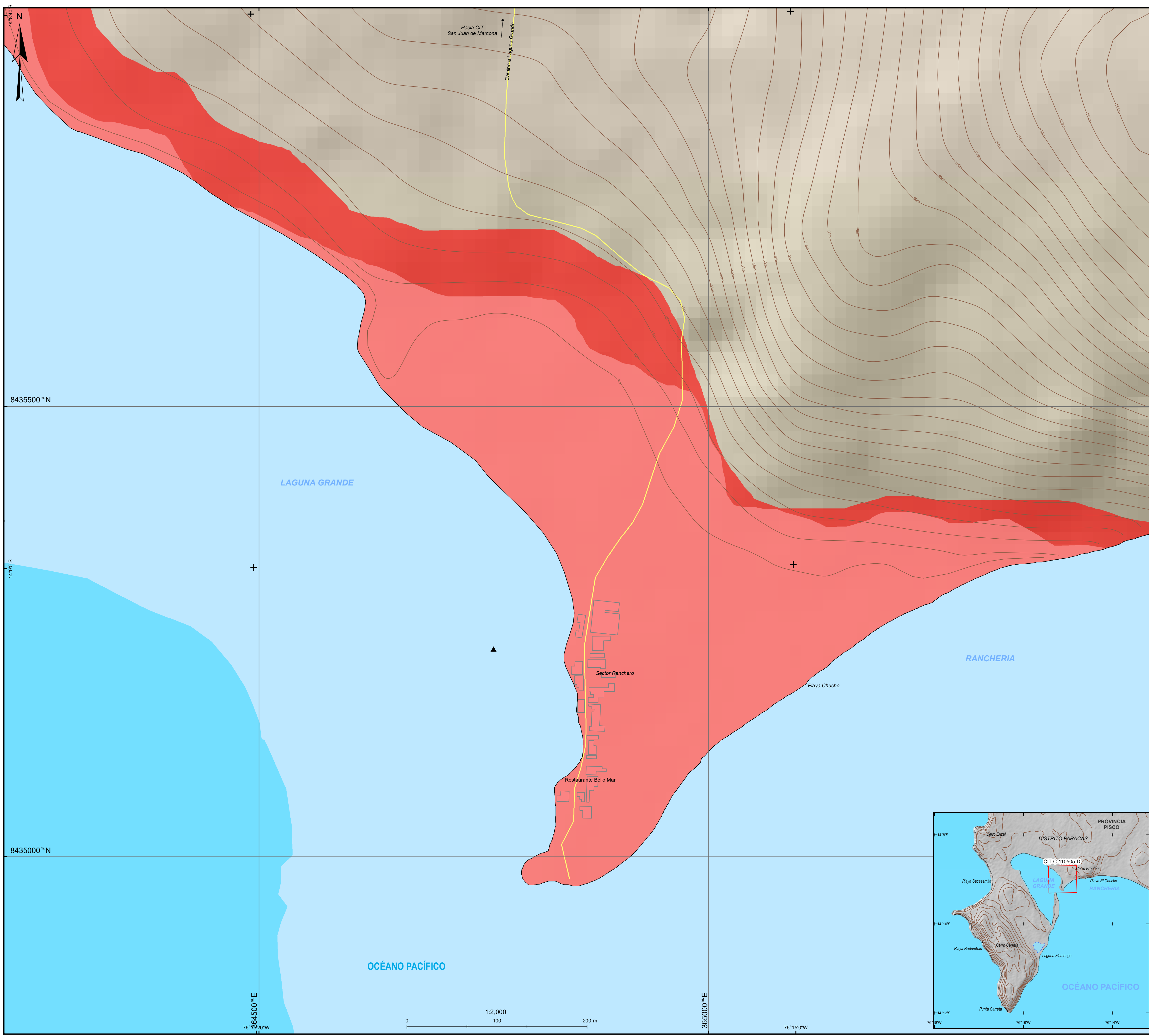
ALTURA DEL TSUNAMI PARA UN EVENTO SÍSMICO DE 9.0 Mw EN EL SECTOR RANCHERO - ICA
