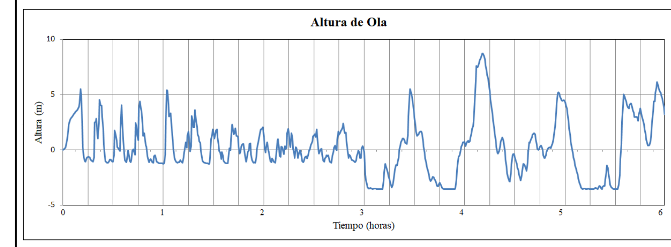
ALTURA DEL TSUNAMI PARA UN EVENTO SÍSMICO DE 9.0 Mw EN EL SECTOR RANCHERO - ICA
