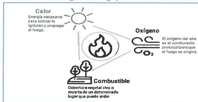
Ilustración 37 Triángulo del fuego para incendios forestales
