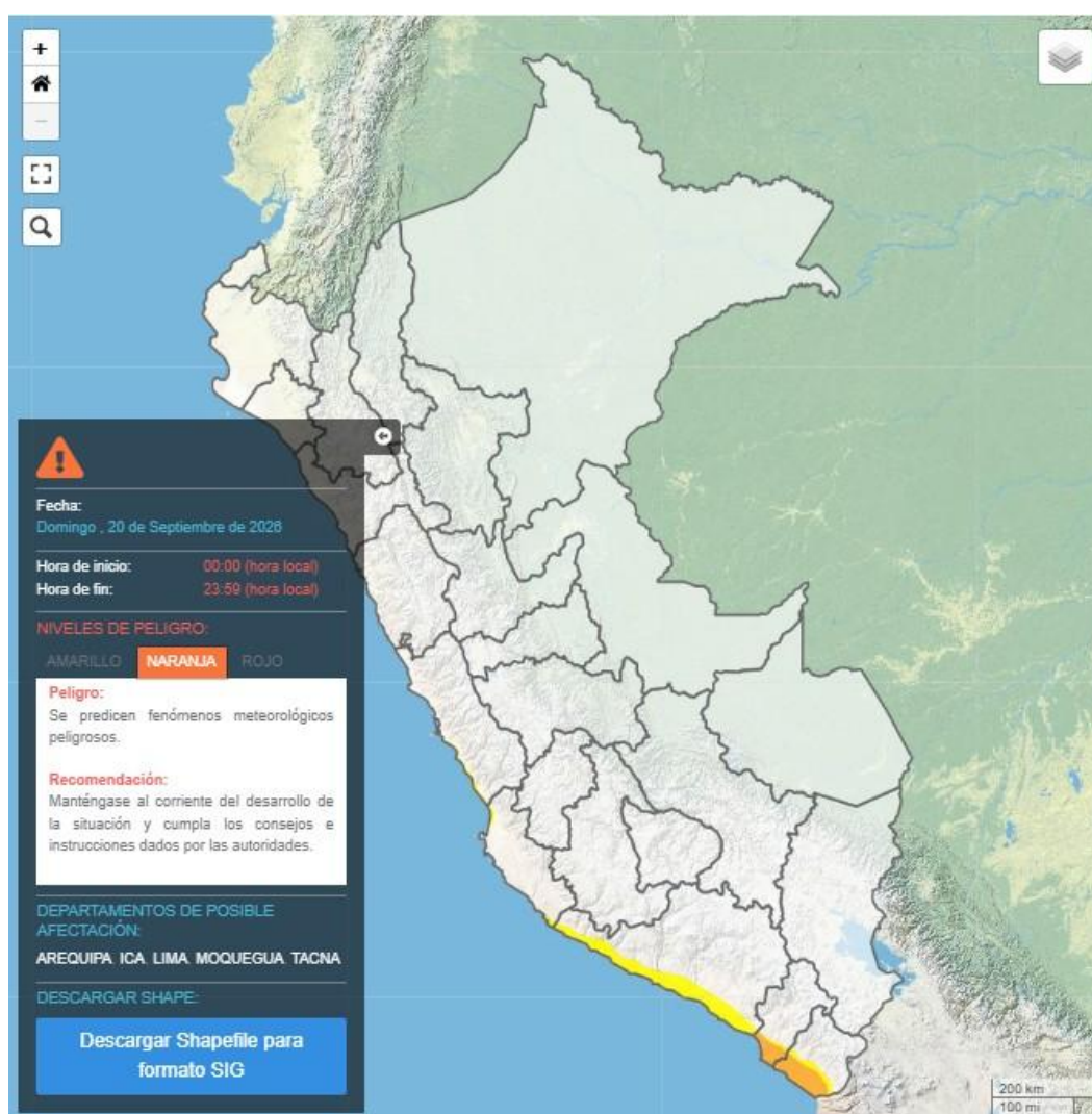
Figura 2. Pronóstico de llovizna en la costa centro y sur del 20 de setiembre del 2026
