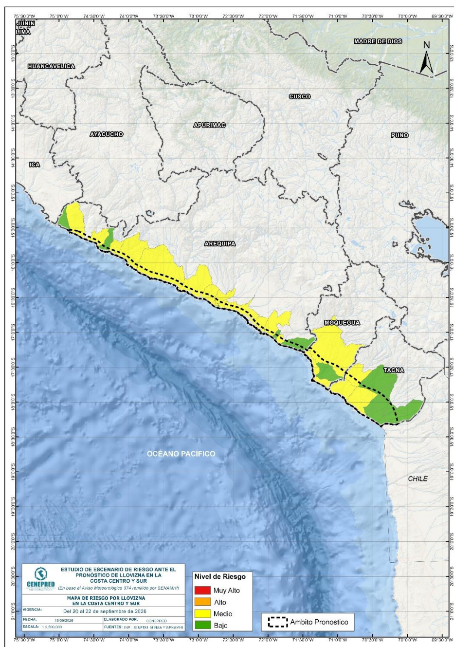
Figura 6. Escenario de riesgo por movimientos en masa según el pronóstico de llovizna en la costa centro y sur
