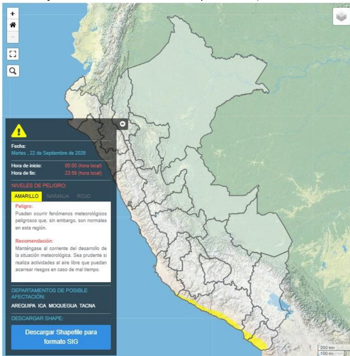
Figura 4. Pronóstico de llovizna en la costa centro y sur del 22 de septiembre del 2026
