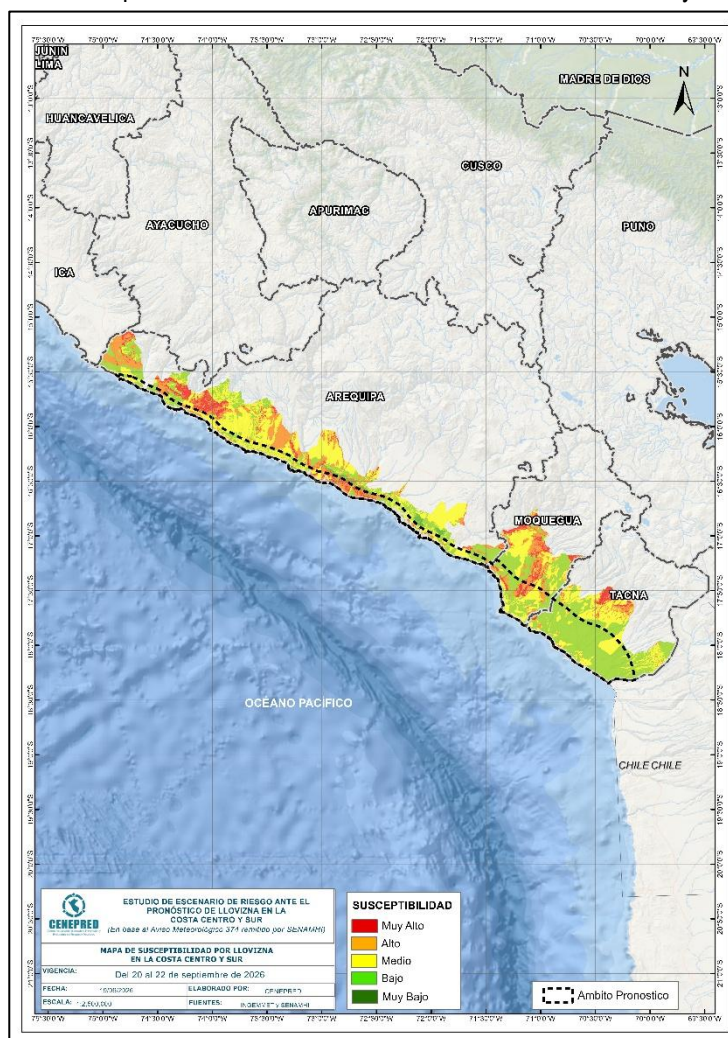
Figura 5. Susceptibilidad a movimientos en masa en la costa centro y sur
