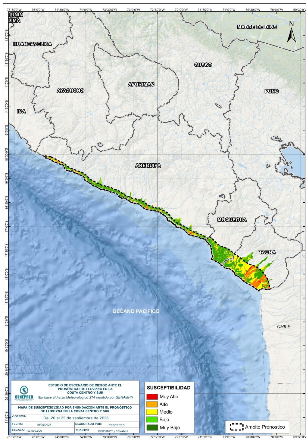
Figura 7. Escenario de riesgo por inundaciones en el ámbito del pronóstico de llovizna en la costa centro y sur del 20 al 22 de septiembre del 2026
