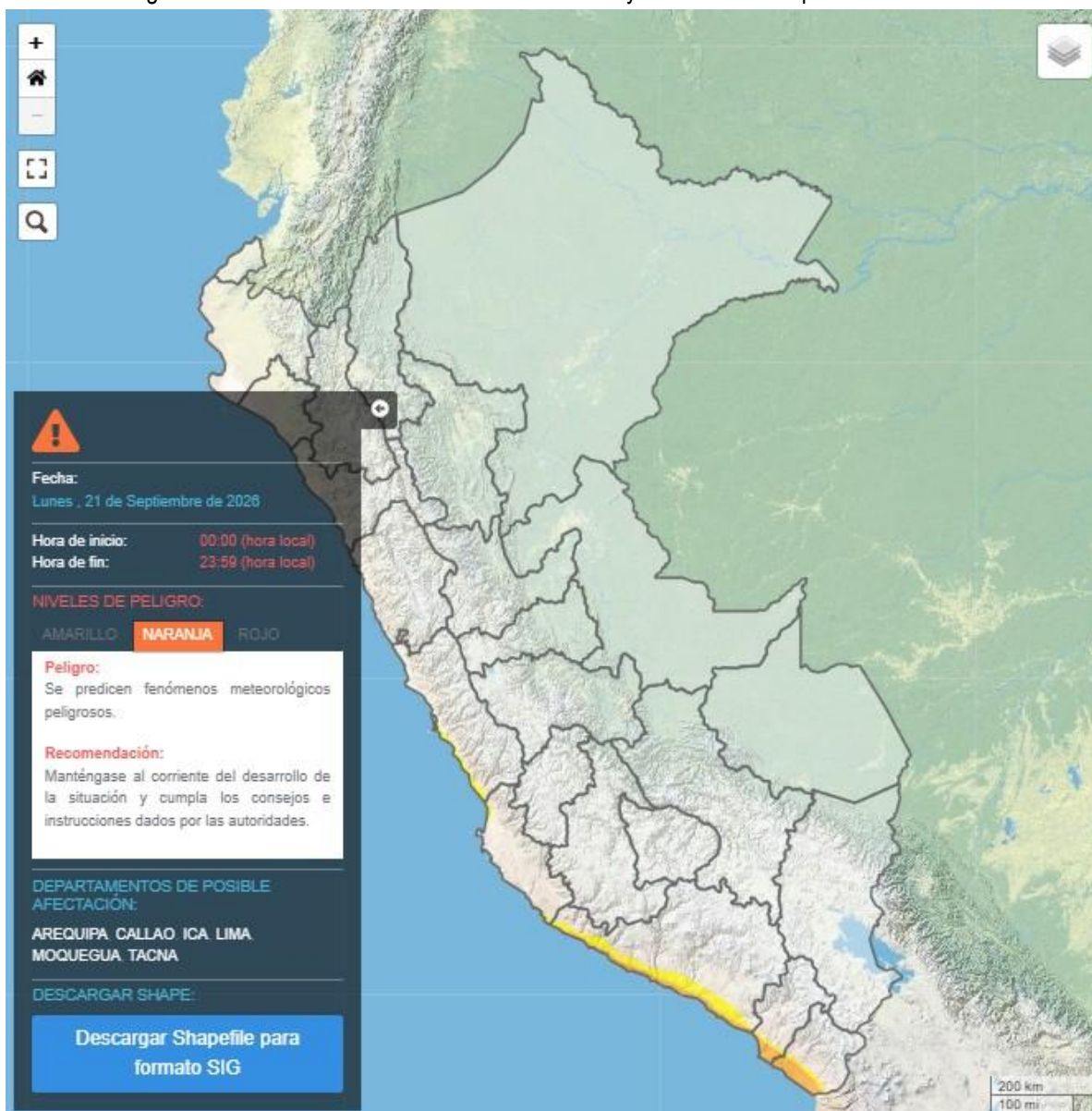
Figura 3. Pronóstico de llovizna en la costa centro y sur del 21 de septiembre del 2026
