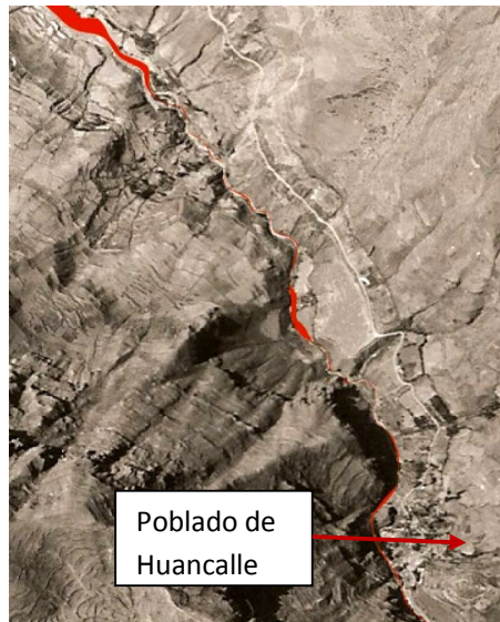
Fig. 10: Sector dos de la parte baja de la quebrada Pinchimayocc.
