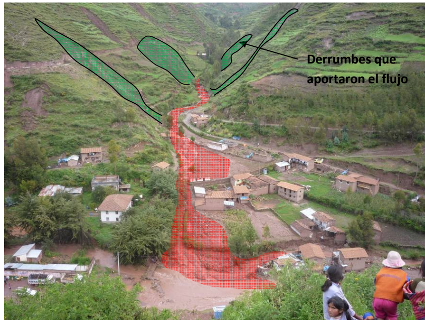
Foto 1: Comunidad Campesina de Ccaccacolla en la confluencia de las quebradas Ccalla Rayan y Pinchimayocc tras el aluvión del 28 de febrero.
