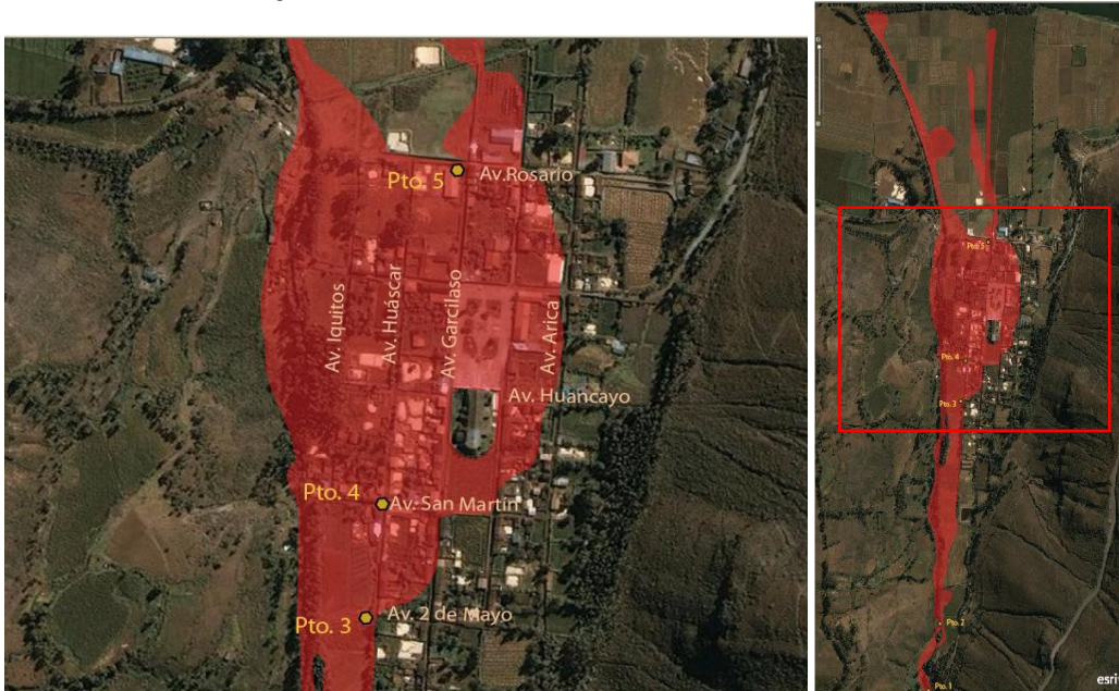
Fig. 13: Recorrido del aluvión del 28 de febrero y 1 de marzo al norte del abanico aluvial de Taray; mostrando su desplazamiento a lo largo de casi todo el poblado.
