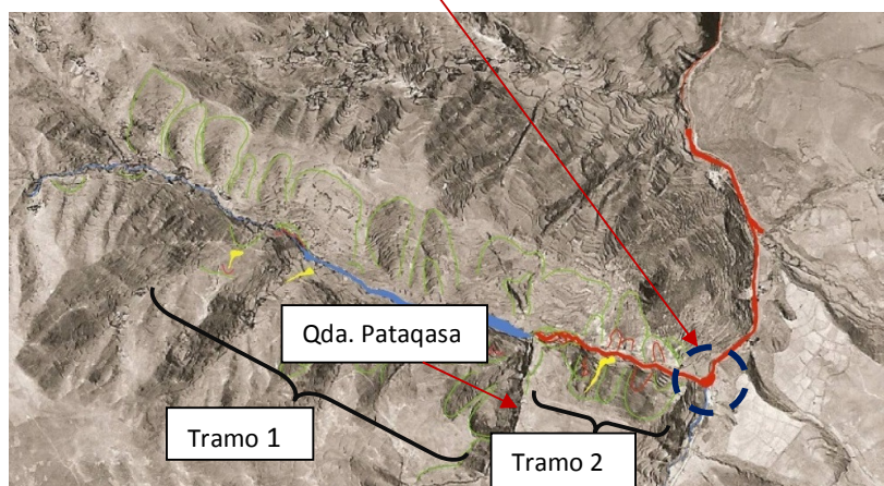
Foto 6 y Fig. 8: Vista del poblado de Ccaccacolla en el tramo 2 de la quebrada Ccalla Rayan el día 1 de marzo.
