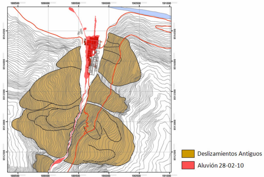
Fig. 6: Grandes deslizamientos antiguos a ambos márgenes en la parte baja de la quebrada Pinchimayoc.
