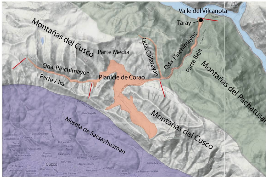
Fig. 4: Mapa geomorfológico local.
