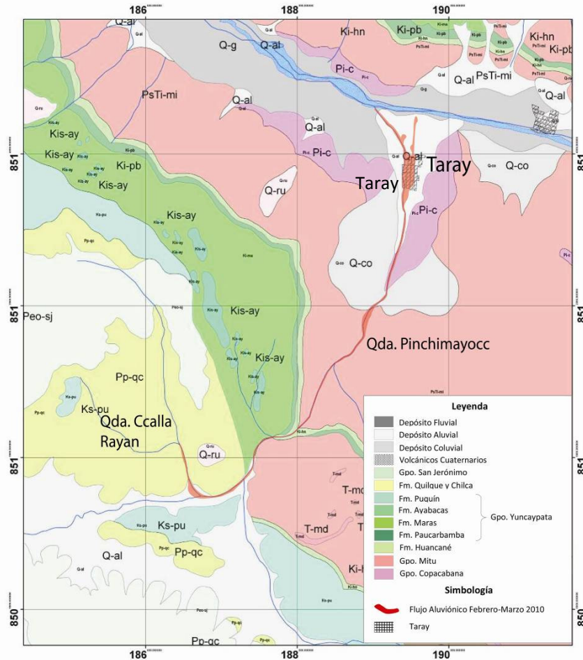
Fig. 5: Mapa geológico del área de estudio.
