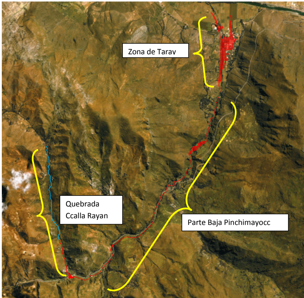
Fig. 2: Ubicación de las quebradas Ccalla Rayan y Pinchimayocc al sur del poblado de Taray. En rojo zonas afectadas por el aluvión. Además se muestran las 3 zonas de estudio en amarillo.
