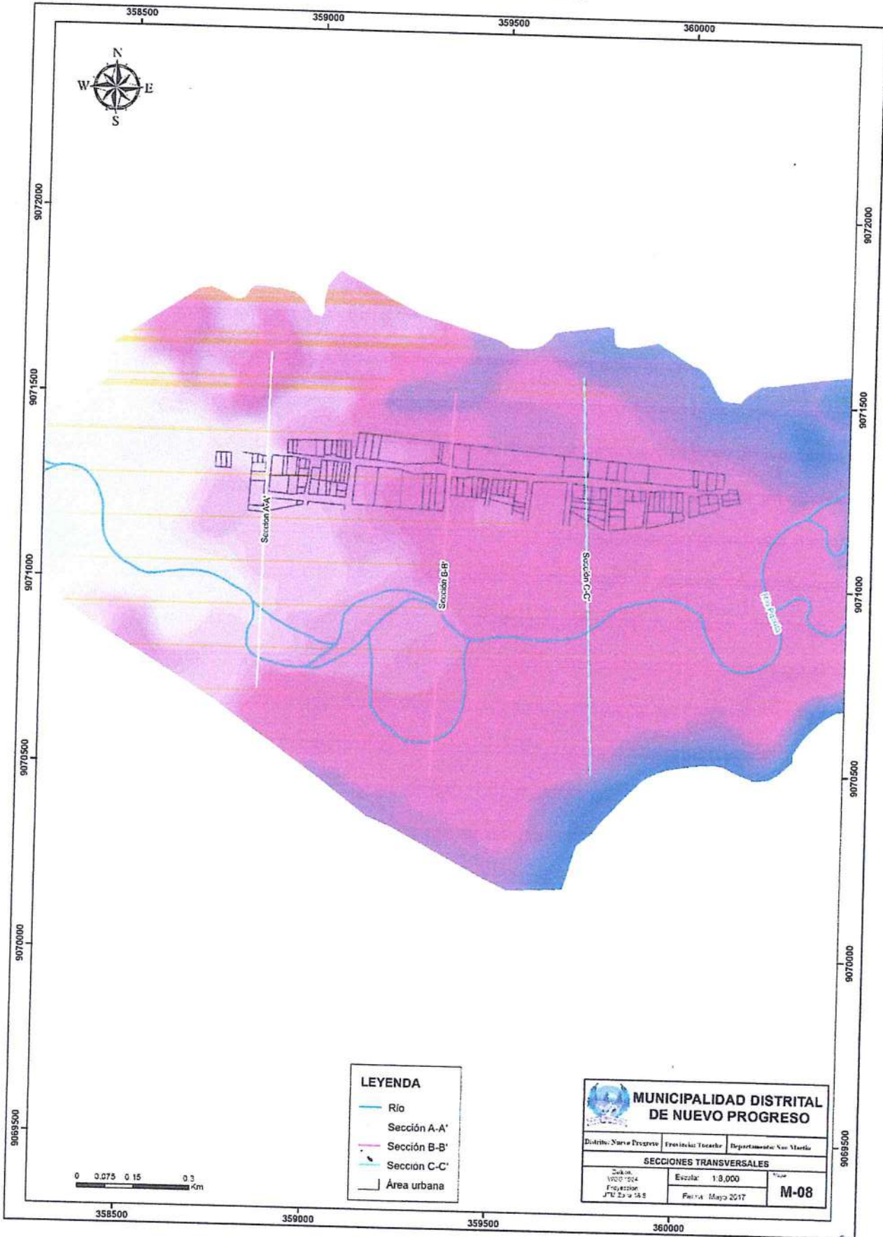
Figura 12: Mapa de ubicación de las secciones transversales de A-A', B-B' y C-C'
