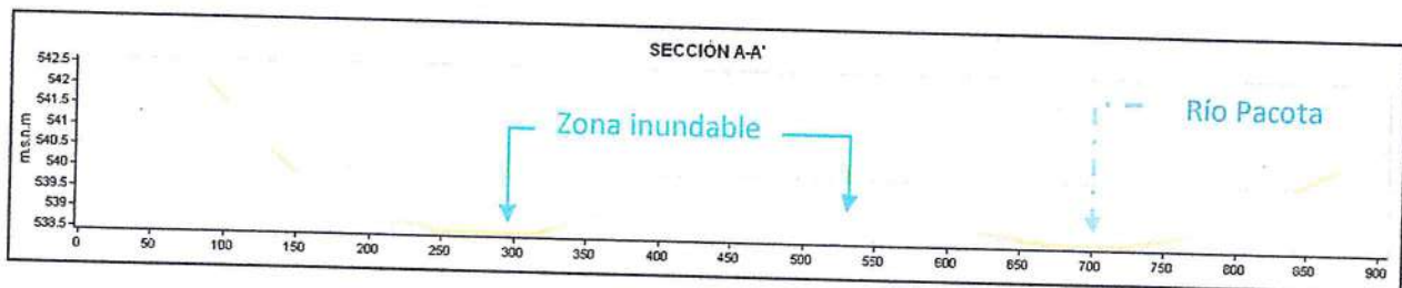
Figura 09. Perfil transversal de la sección A-A'
