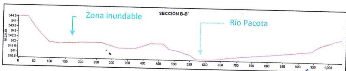
Figura 10. Perfil transversal de la sección B-B'
