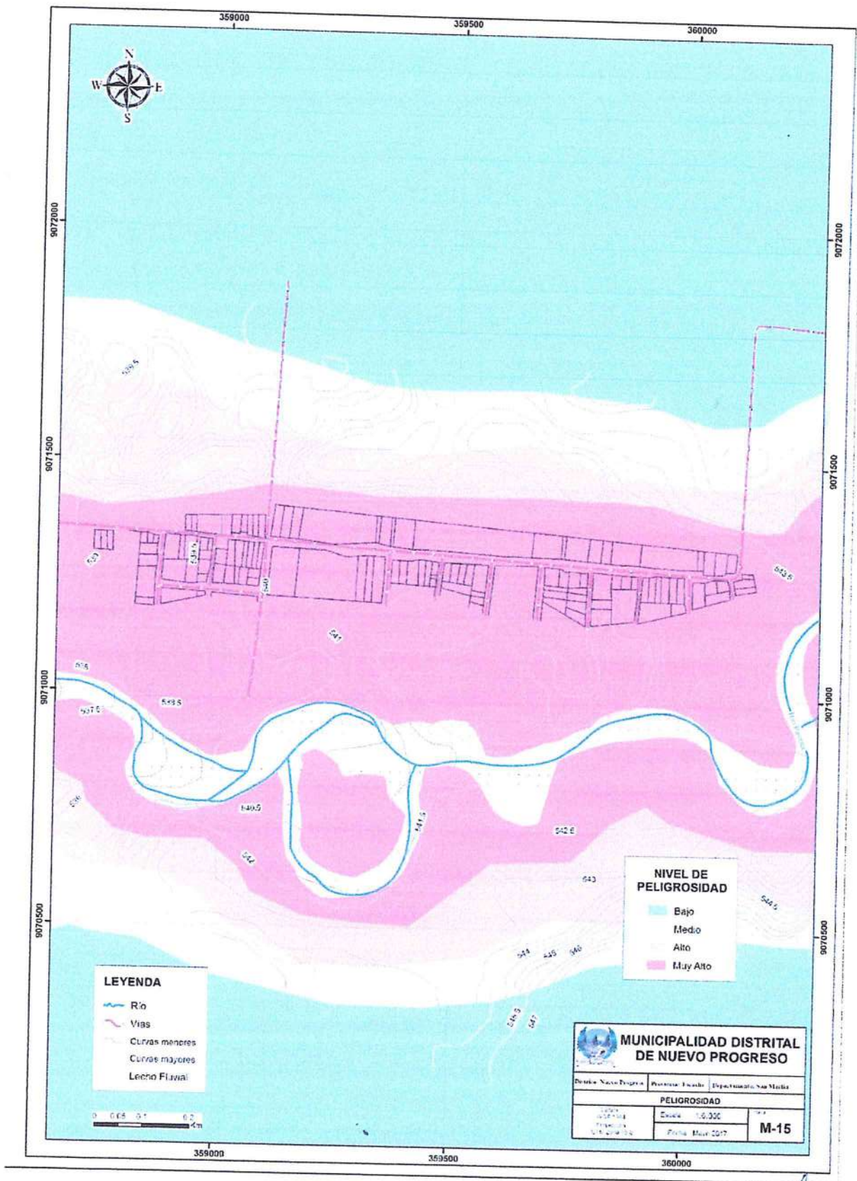
Figura 20: Mapa de peligro de la localidad de Pacota
