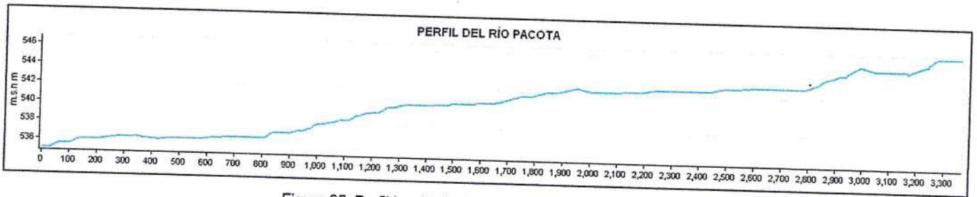
Figura 05: Perfil longitudinal del río en la localidad de Pacota.
