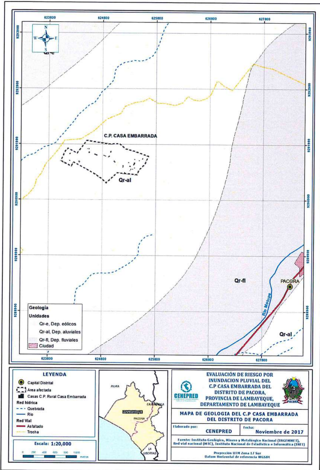
Figura N° 04 – Mapa Geológico
