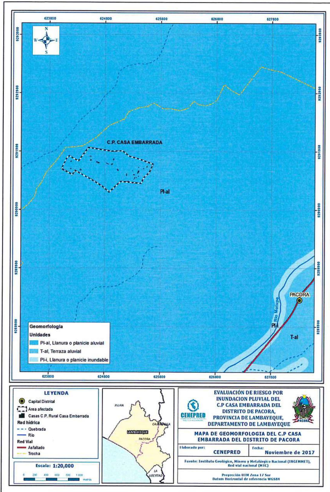
Figura N° 03 – Mapa Geomorfológico
