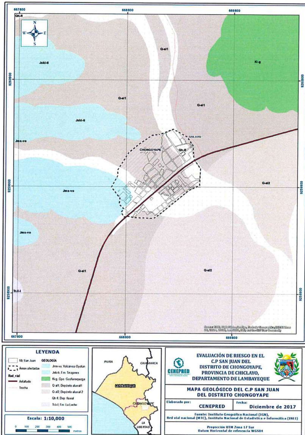
Figura N° 04 – Mapa Geológico
