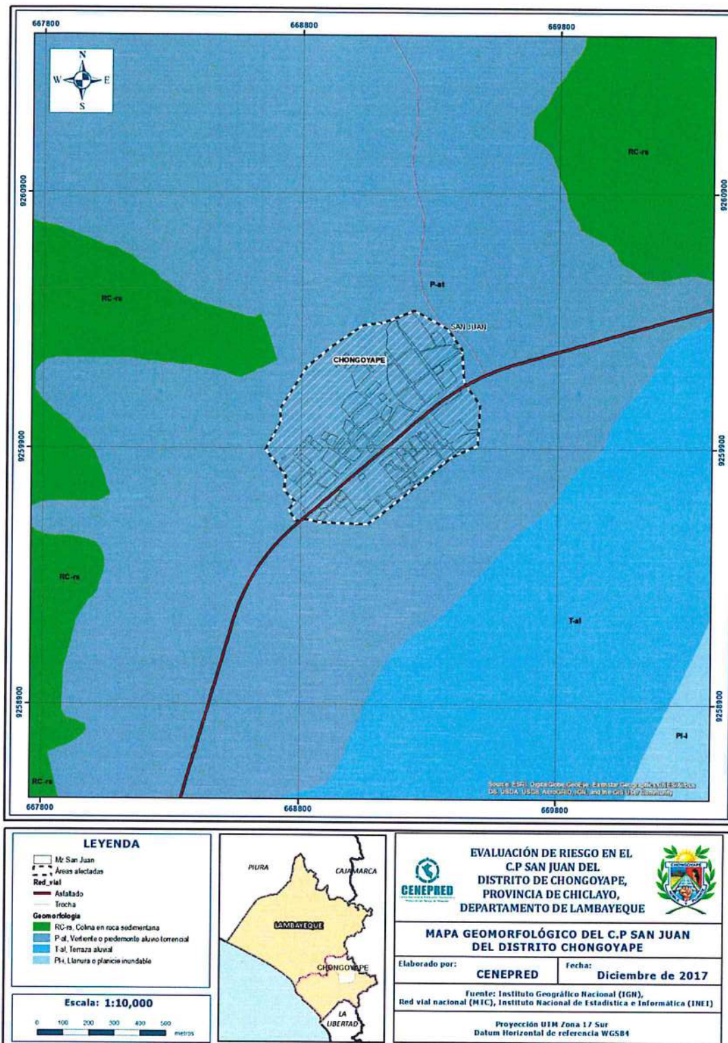
Figura N° 03 – Mapa Geomorfológico
