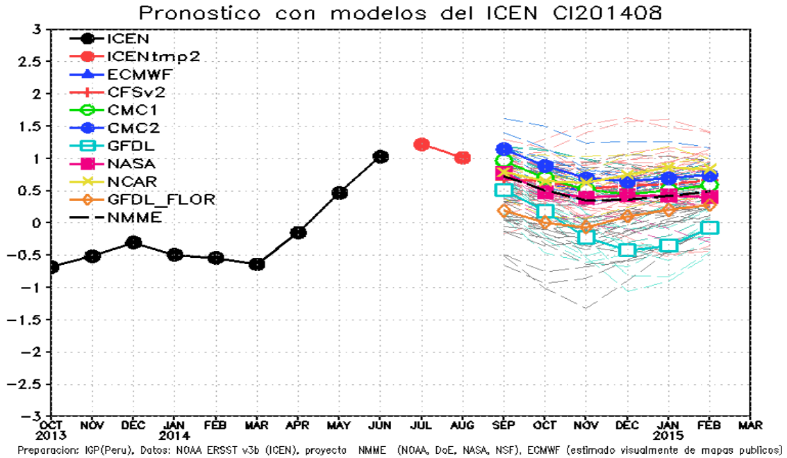
Figura 5. Índice Costero El Niño (ICEN, negro con círculos llenos) y sus valores temporales (ICENtmp, rojo con círculo lleno). Además, pronósticos numéricos del ICEN (media móvil de 3 meses de las anomalías pronosticadas de TSM en Niño 1+2) por diferentes modelos climáticos. Las líneas entrecortadas corresponden a los miembros de los "ensembles". Los pronósticos de los modelos CFSv2, CMC1, CMC2, GFDL, NAS y GFDL_FLOR tienen como condición inicial el mes de agosto de 2014. El modelo ECMWF tiene como condición inicial el mes de agosto de 2014. (Fuente: IGP, NOAA, proyecto NMME, ECMWF).
