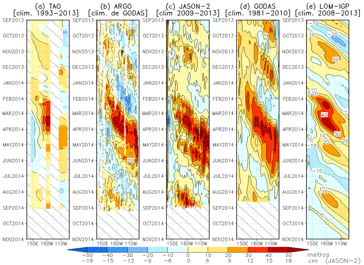
Figura 10. Diagrama longitud-tiempo a lo largo de la línea ecuatorial de la anomalía de la profundidad de la isoterma de 20°C (a, b, d y e) y del nivel del mar (c). Los datos son de a) las boyas TAO/TRITON, b) los derivadores Argo, c) el altímetro satelital JASON-2, d) el sistema de asimilación de datos GODAS, y e) el modelo LOM-IGP (forzado por ASCAT, y \tau_{\text{aux}}=0 para el pronóstico). Las líneas diagonales representan una propagación hacia el este con velocidad de 2.6 m/s. (Elaboración: IGP)
