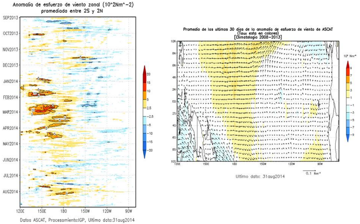
Figura 13. Izquierda: Diagrama longitud-tiempo de las anomalías de esfuerzo de viento zonal ecuatorial basado en datos del escaterómetro ASCAT. Derecha: Mapa del promedio de 30 días, hasta el 31 de agosto de 2014, incluyendo los vectores de esfuerzo zonal. (Elaboración: IGP)
