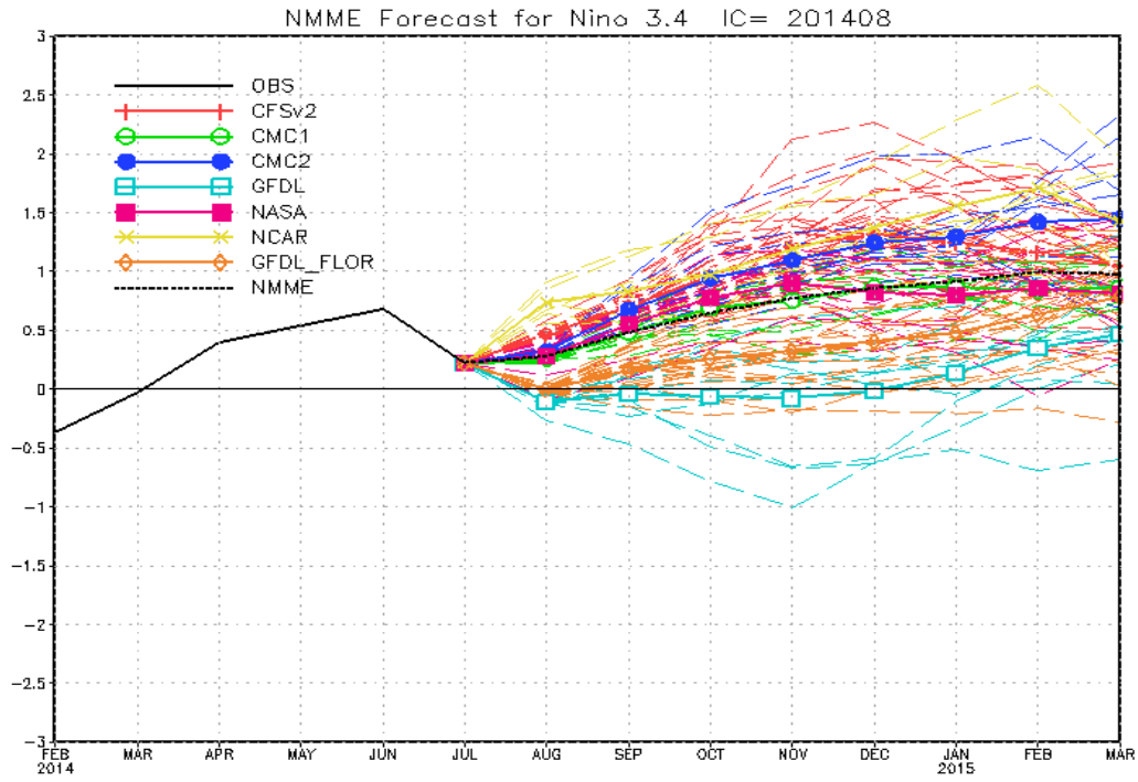
Figura 6. Similar a Fig. 6 pero para el índice Niño 3.4 mensual observado y pronosticado por los modelos de NMME. (Fuente: http://www.cpc.ncep.noaa.gov/products/NMME/ )
