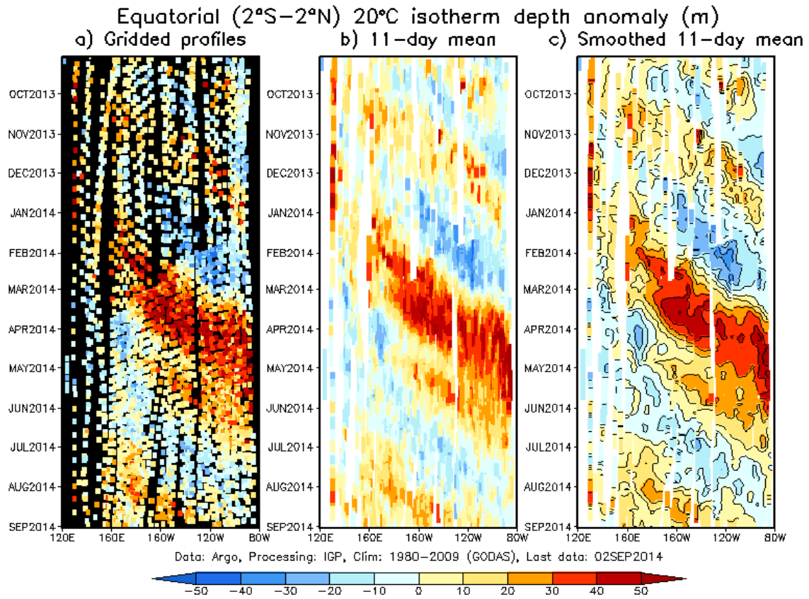
Figura 12. Diagrama longitud-tiempo de las anomalías de la profundidad de la isoterma de 20C ecuatorial de derivadores Argo. a) Perfiles individuales grillados, b) media móvil de 11 días, c) versión suavizada de b). (Elaboración: IGP)
