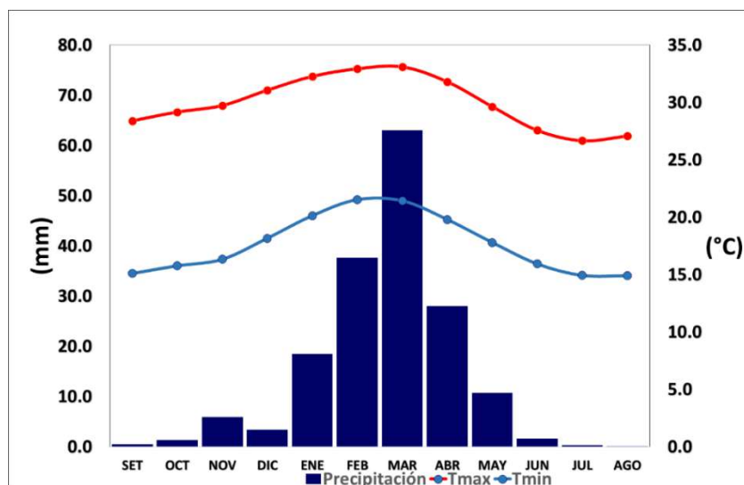
Gráfico N° 11 - Comportamiento temporal de la temperatura del aire y precipitación promedio en la estación meteorológica Jayanca
