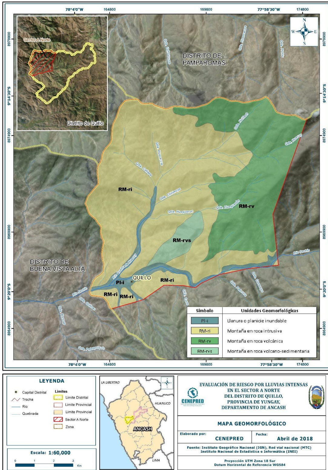
Figura 08. Mapa Geomorfológico
