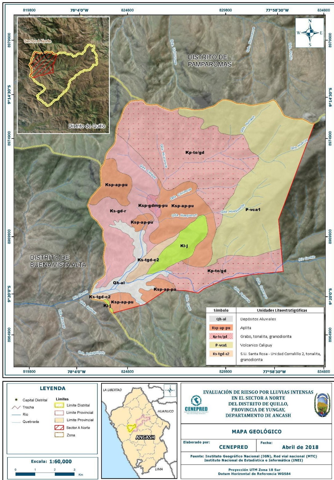
Figura 09. Mapa Geológico
