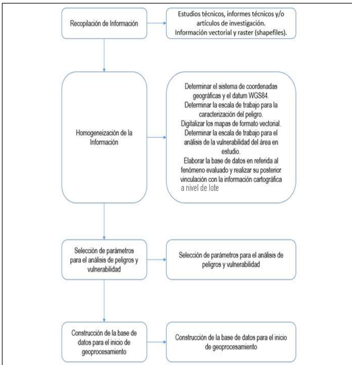
Gráfico N° 11: Flujograma general del proceso de análisis de información
