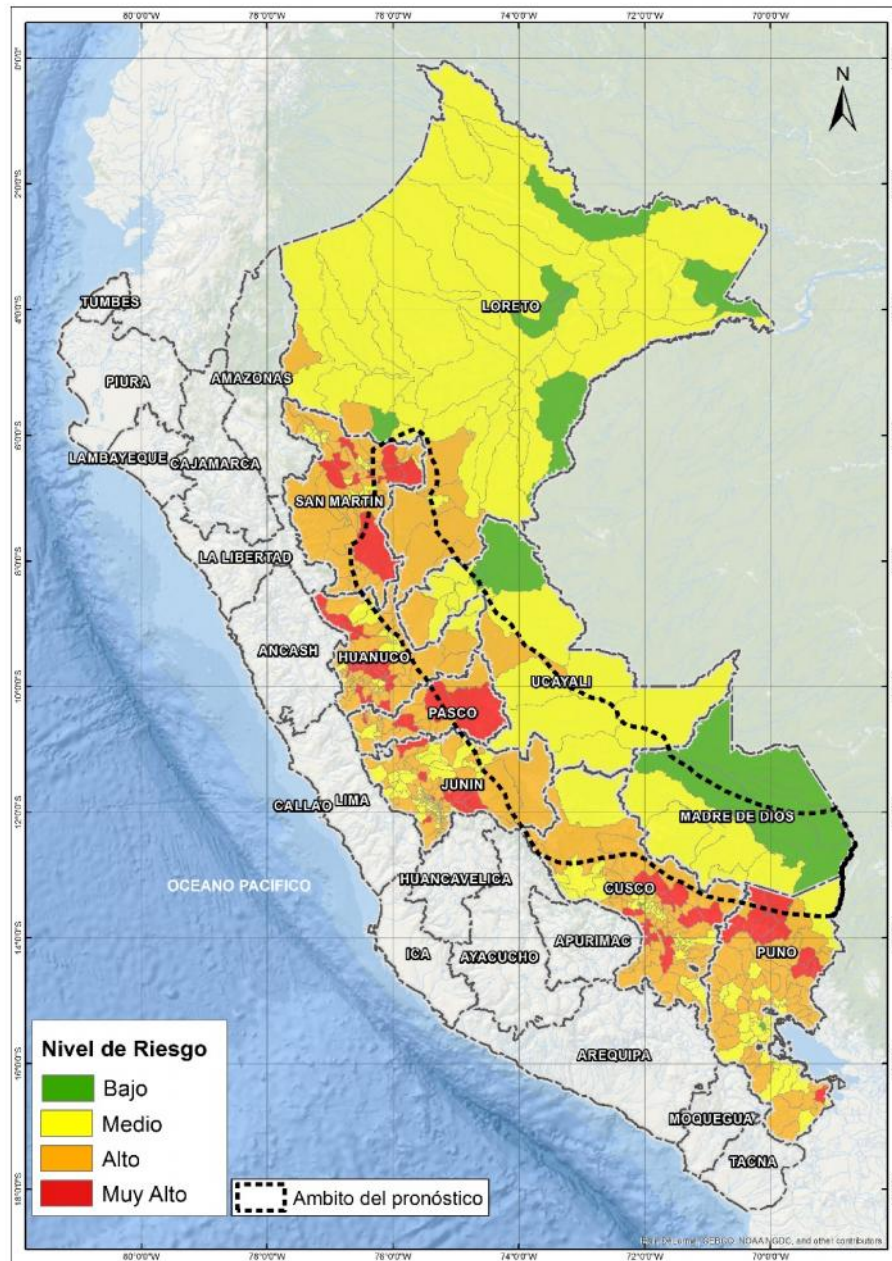
Figura 4. Escenario de riesgo por movimientos en masa en base al pronóstico de precipitación para el periodo del 07 al 09 de enero de 2019
