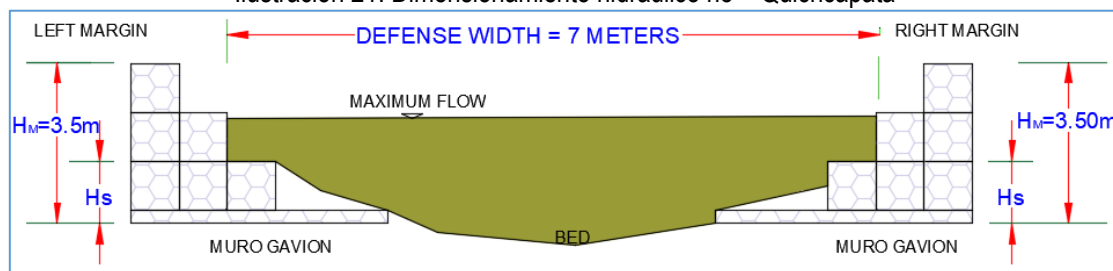
Ilustración 21: Dimensionamiento hidráulico río – Quichcapata
