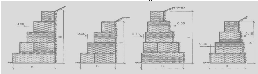
Ilustración 17: muro de gaviones
