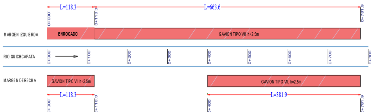
Ilustración 22: Planteamiento hidráulico de control de inundación río – Quichcapata
