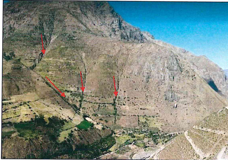
Figura 11: Cárcavas de fuerte pendiente, con cauces en forma de V, confluyendo hacia la quebrada que cruza la zona media del área evaluada.
