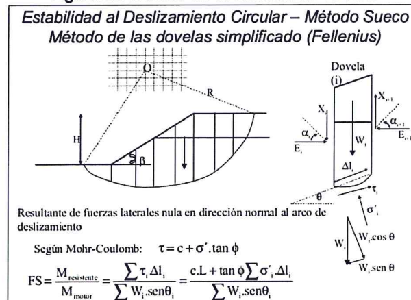
Figura 24: Modelo de deslizamiento circular
