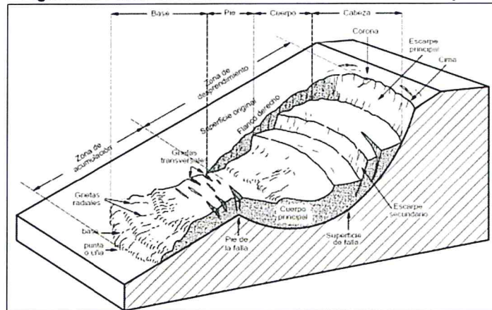
Figura 23: Parámetros de un deslizamiento rotacional típico
