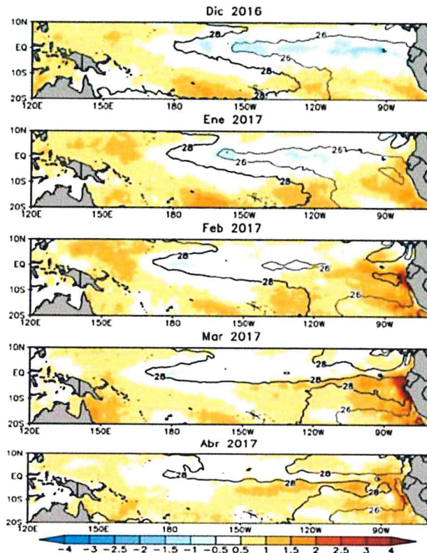
Gráfico N° 08. Anomalía de la Temperatura superficial del mar (°C) en el Pacífico ecuatorial para el periodo diciembre 2016 – abril 2017
