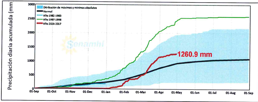
Gráfico N° 09. Precipitación diaria acumulada en la estación meteorológica Niepos
