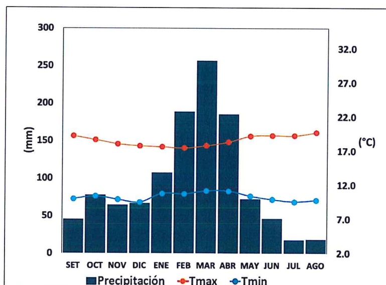
Gráfico N° 07. Comportamiento temporal de la temperatura del aire y precipitación promedio en la estación meteorológica Niepos
