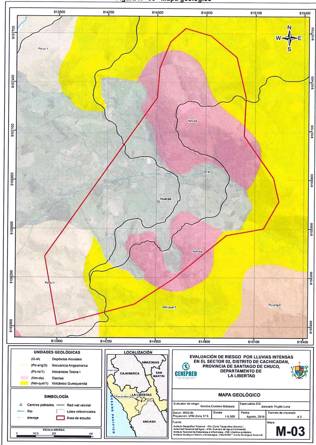
Figura N° 03- Mapa geológico
