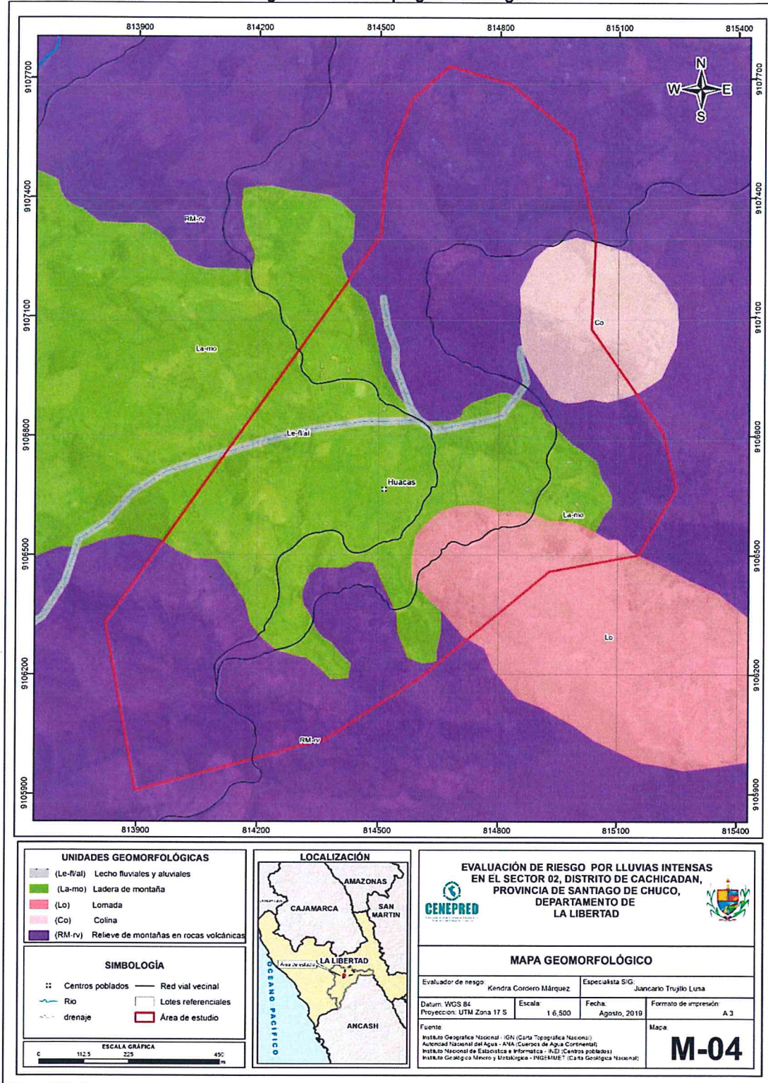
Figura N° 04 – Mapa geomorfológico
