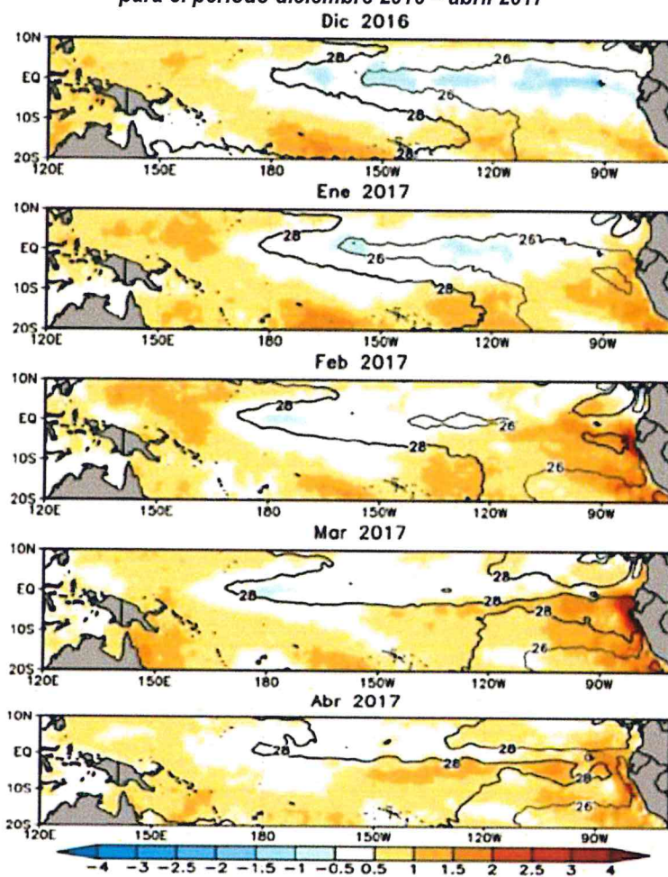
Gráfico 6. Anomalía de la Temperatura superficial del mar (°C) en el Pacífico ecuatorial para el periodo diciembre 2016 – abril 2017
