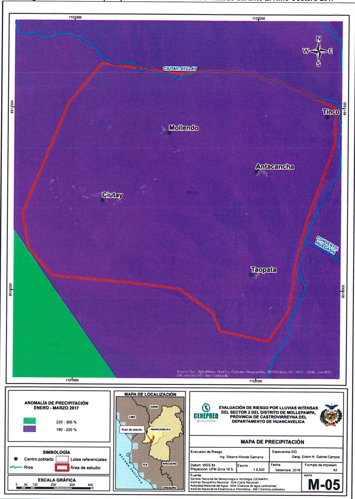
Figura 5. Anomalía de precipitación del mes de enero - marzo durante El Niño Costero 2017
