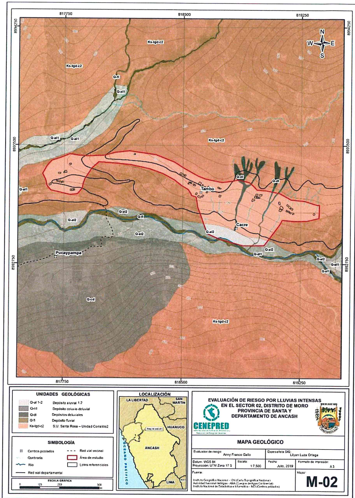
Figura 02: Mapa geológico del Sector 2
