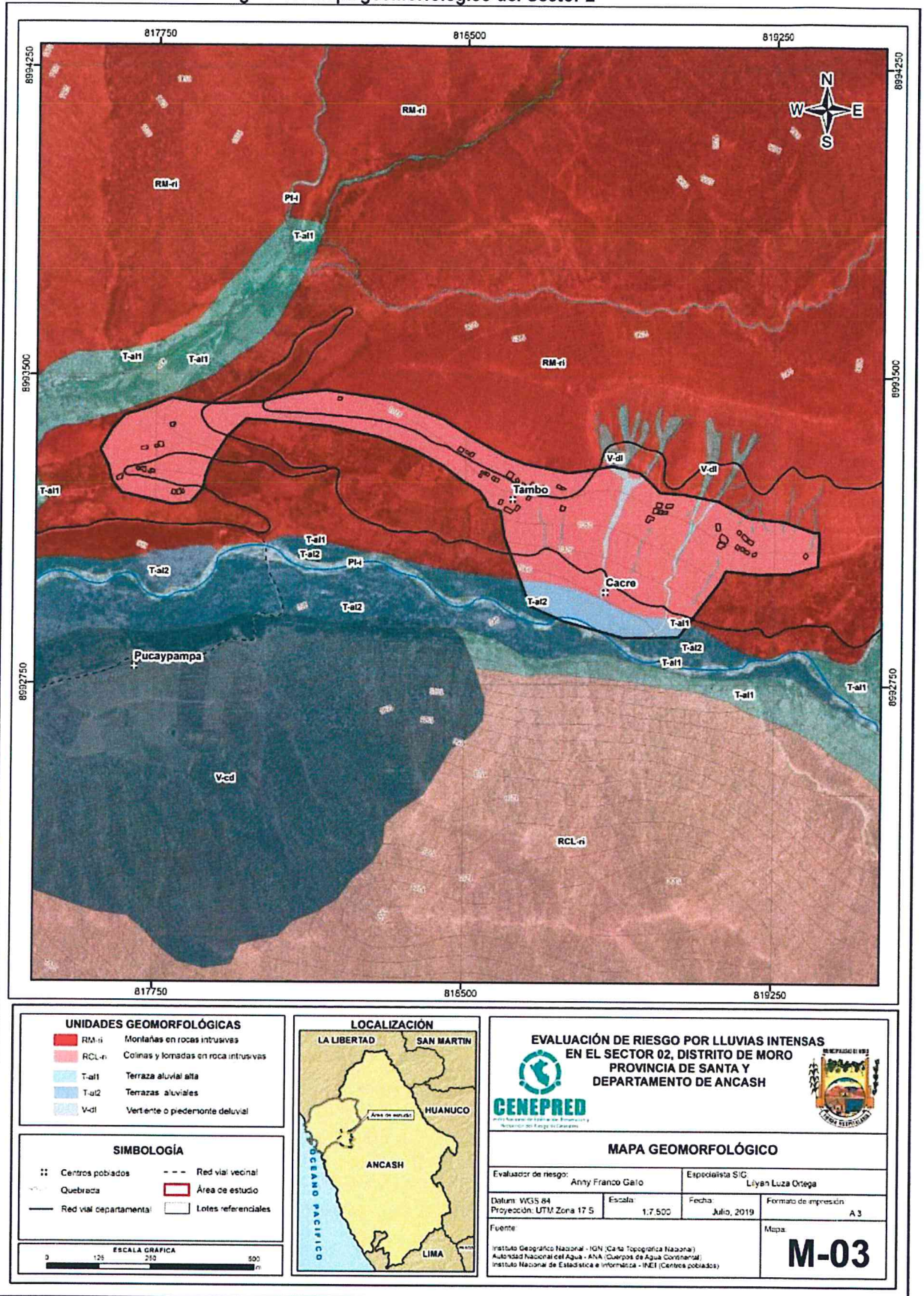
Figura 03: Mapa geomorfológico del Sector 2
