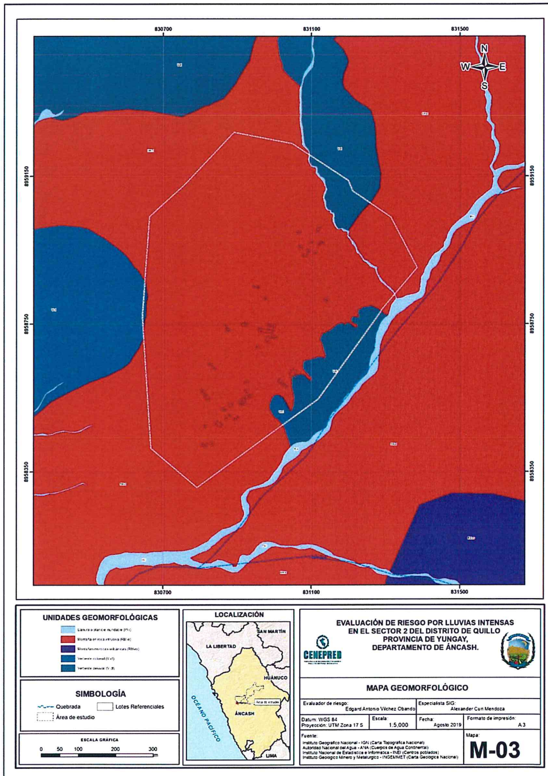
Figura 03. Mapa de Geomorfología del Sector 02 del distrito de Quillo, provincia de Yungay, departamento de Ancash
