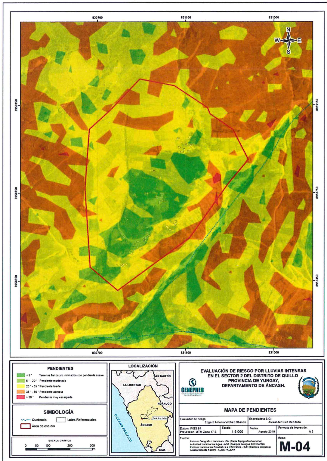
Figura 04. Mapa de Pendientes del Sector 02 del distrito de Quillo, provincia de Yungay, departamento de Ancash
