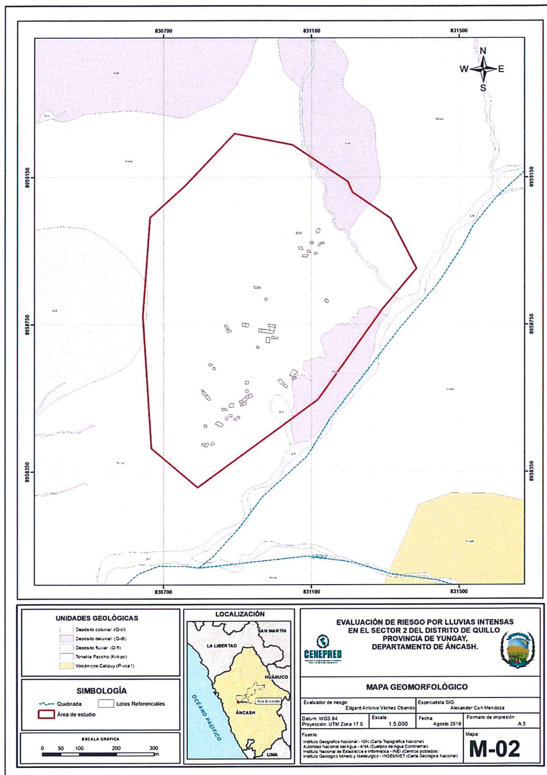
Figura 02. Mapa de Geología del Sector 02 del distrito de Quillo, provincia de Yungay, departamento de Ancash
