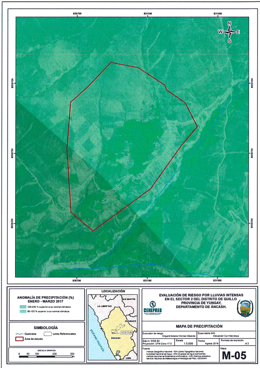
Figura 05. Mapa de Anomalías de lluvias durante El Niño Costero 2017 (Enero-Marzo) para el Sector 02 del distrito de Quillo, provincia de Yungay, departamento de Ancash
