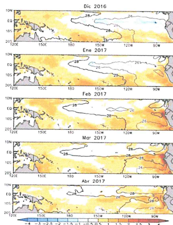
Gráfico N° 09. Anomalia de la Temperatura superficial del mar (°C) en el Pacifico ecuatorial para el periodo diciembre 2016 – abril 2017
