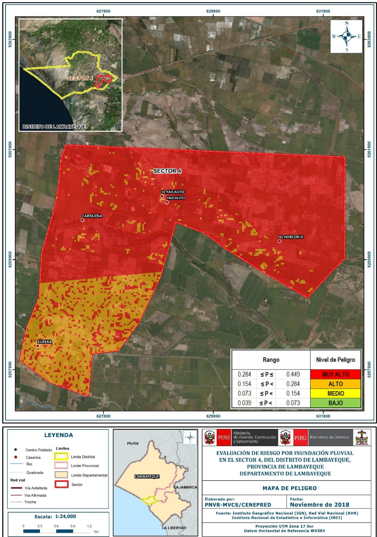
Figura 07: Mapa de peligro por inundación pluvial del Sector 4
