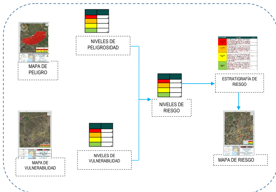
Gráfico N° 6: Flujograma para estimar los niveles de riesgo
