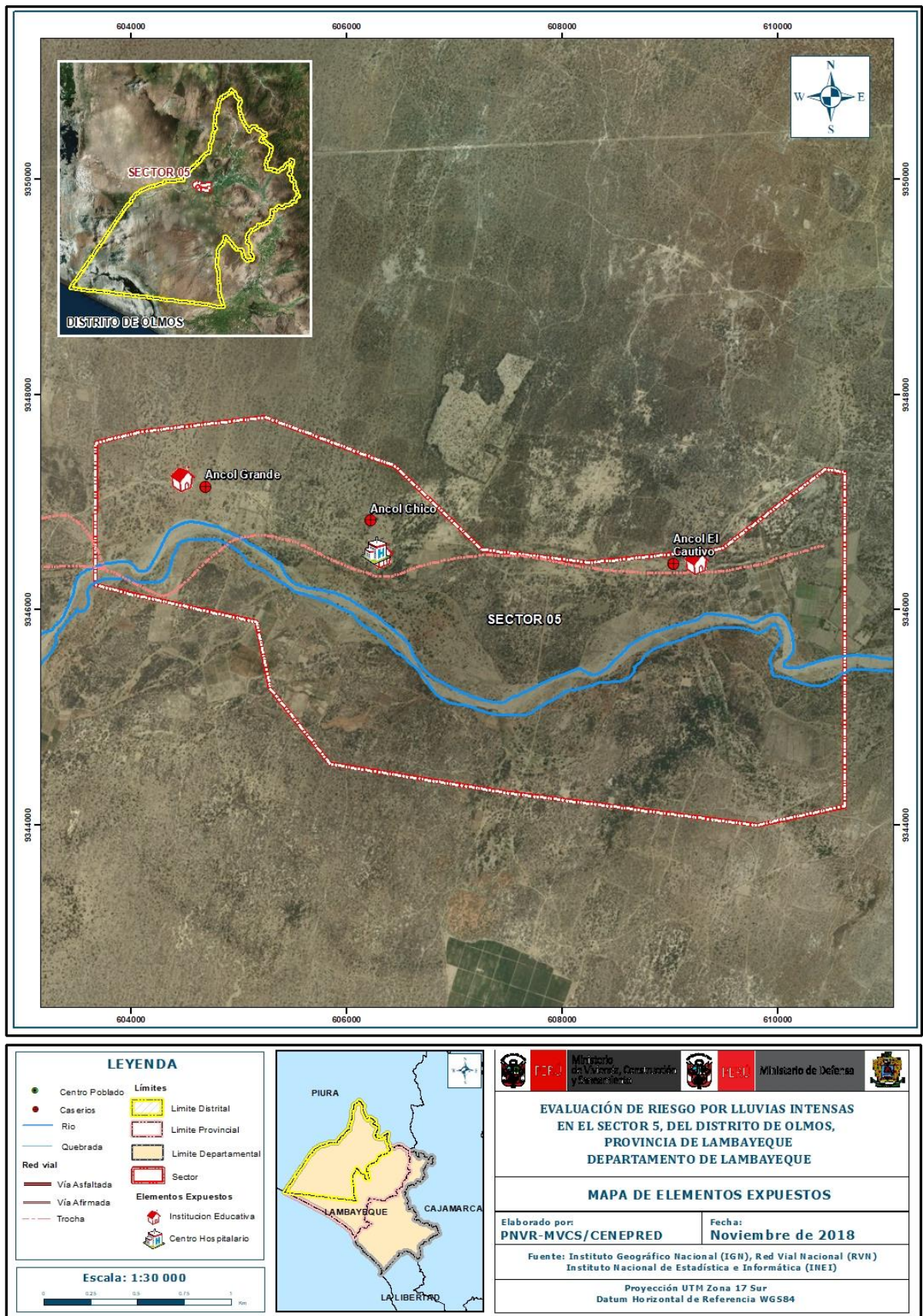
Figura 8: Mapa de elementos expuestos del Sector 5, distrito de Olmos.
