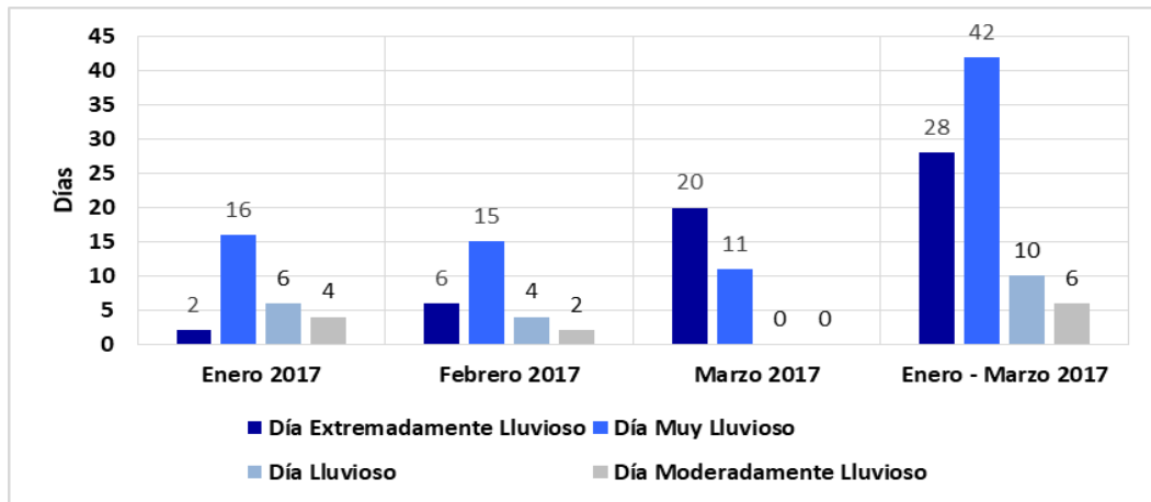
Gráfico N° 2: Frecuencia promedio de lluvias extremas durante El Niño Costero 2017 en el distrito Olmos.
