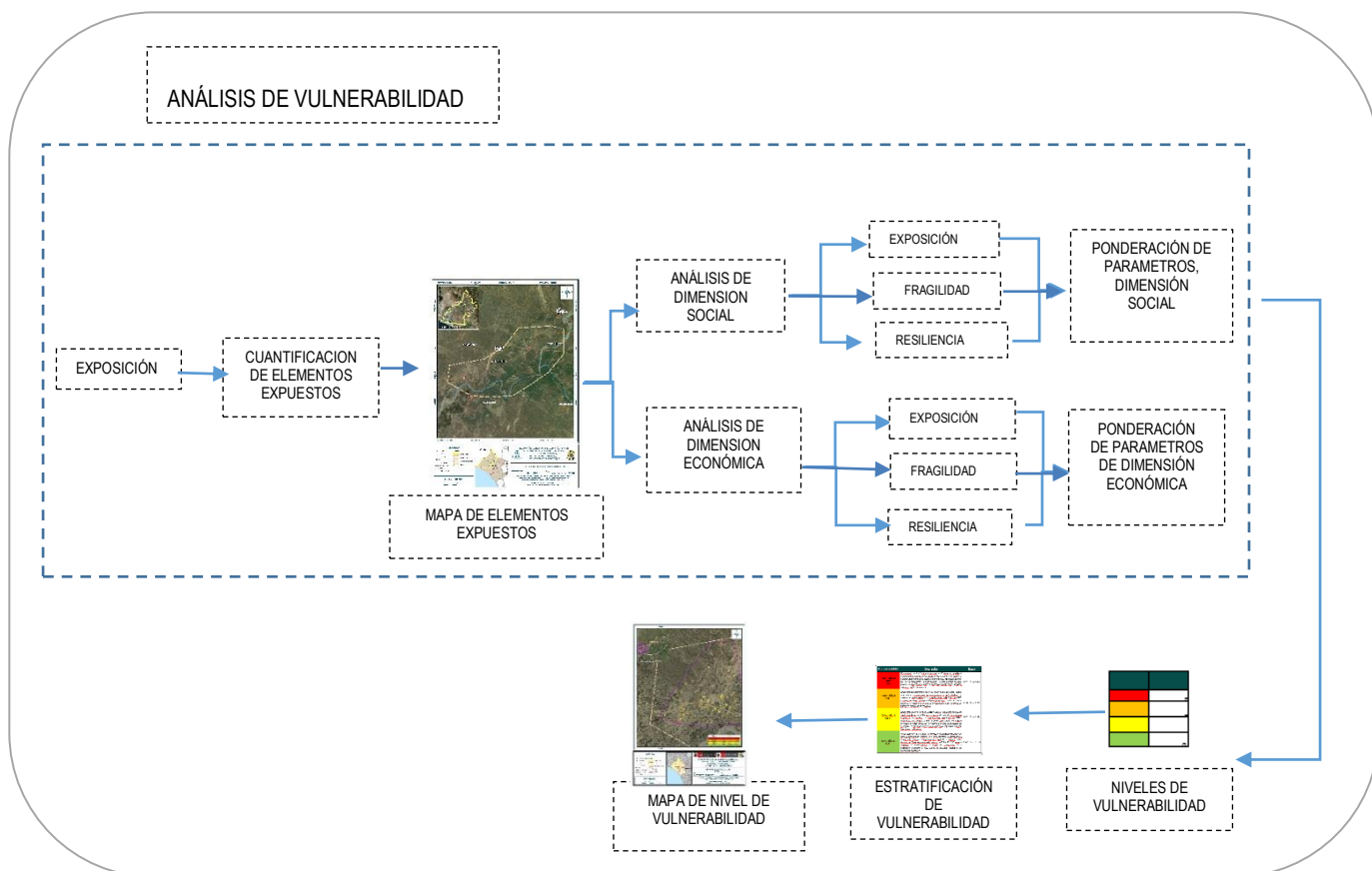
Gráfico N° 5: Metodología para análisis de vulnerabilidad
