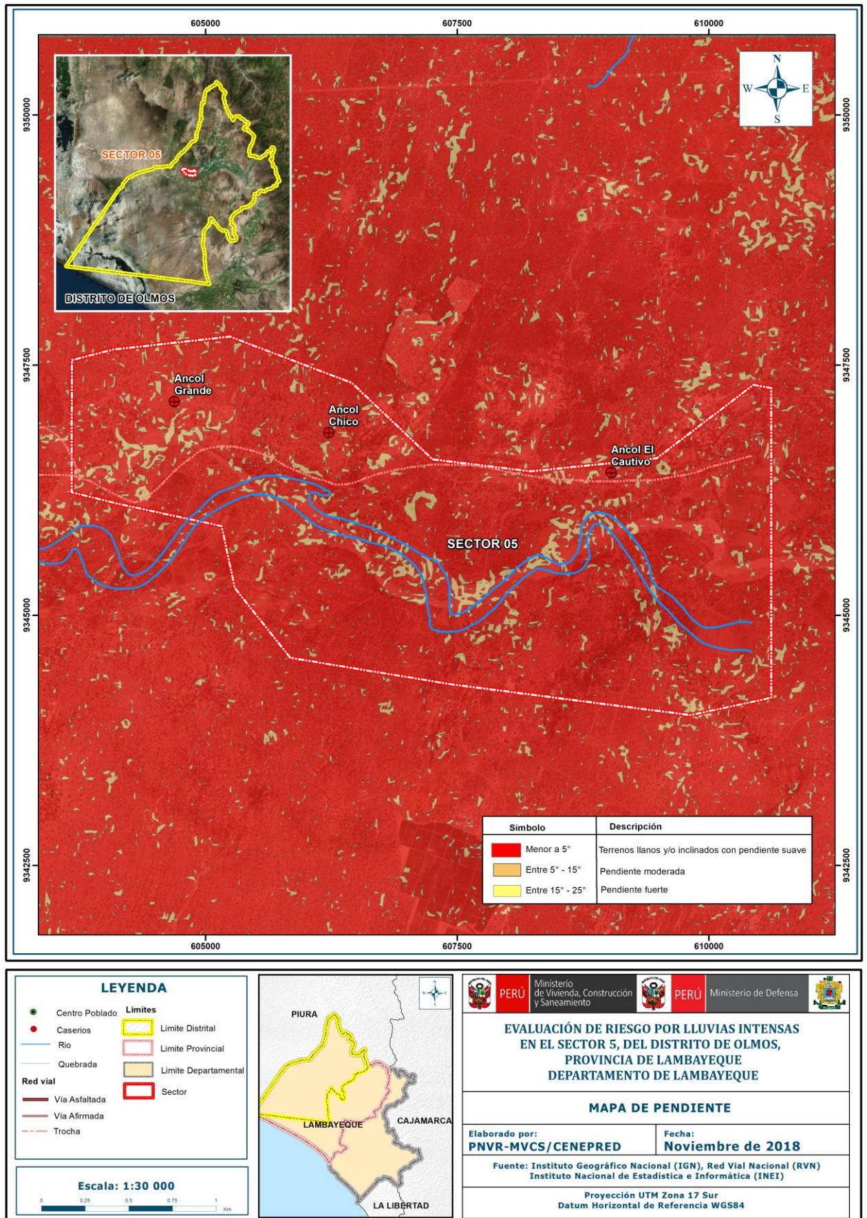
Figura 4: Mapa de Pendiente del Sector 5
