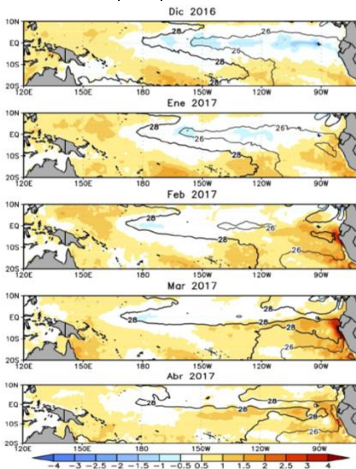
Figura 5: Anomalía de la Temperatura superficial del mar (°C) en el Pacífico ecuatorial para el periodo diciembre 2016 – abril 2017
