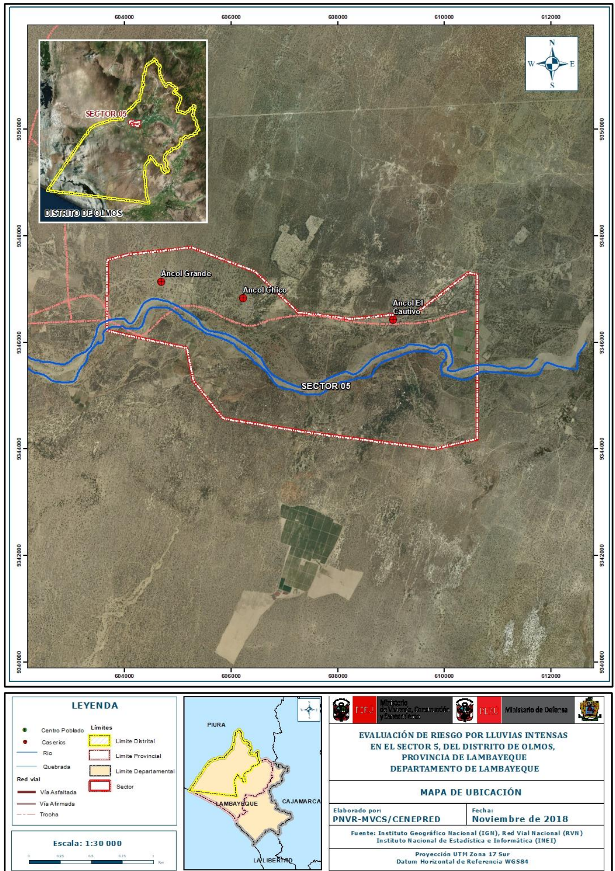
Figura 1: Mapa de Ubicación del Sector 5 del distrito de Olmos
