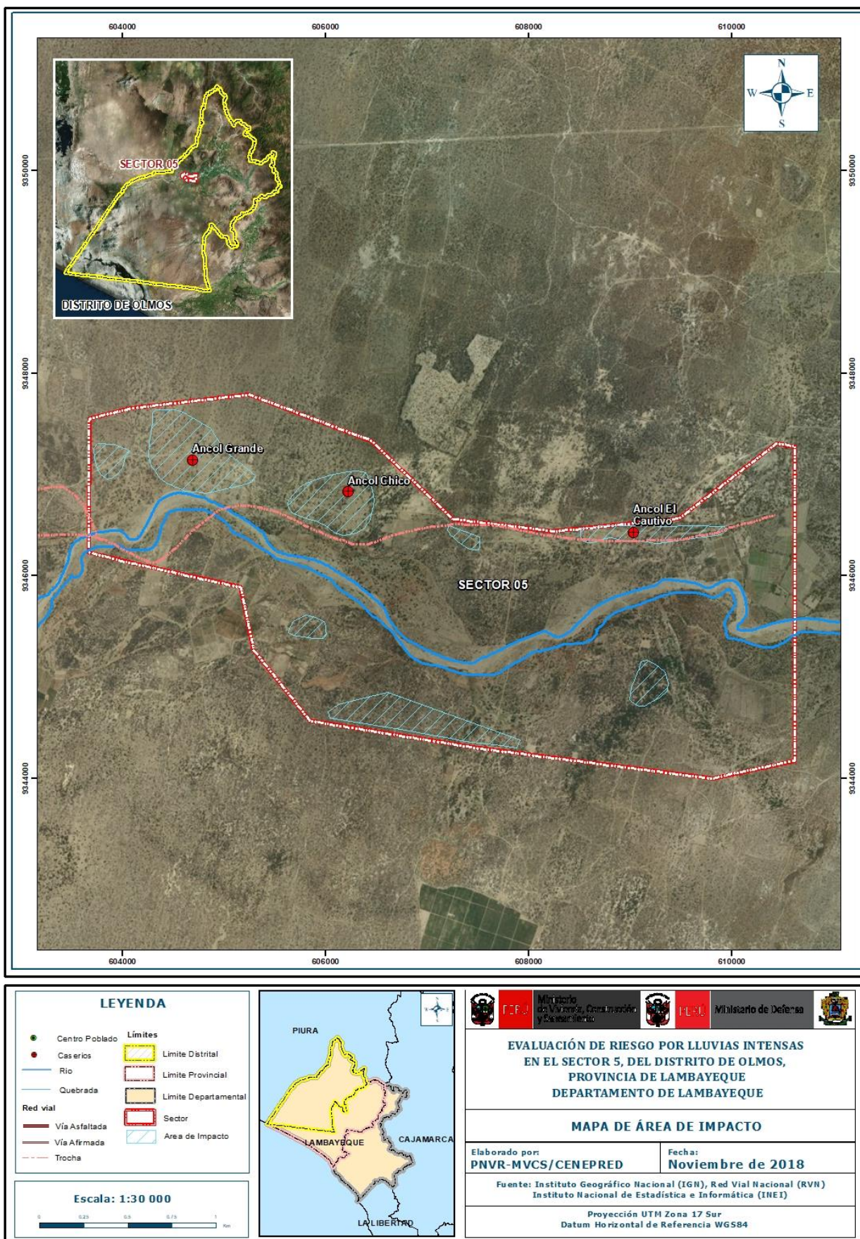
Figura 9: Mapa de Área de Impacto - Sector 5
