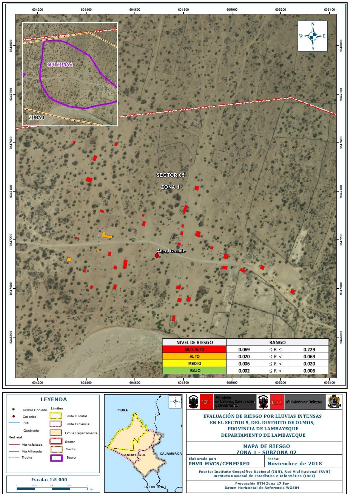
Figura 22: Mapa de Riesgo del Sector 5, distrito de Olmos – Zona 1-Sub Zona 02
