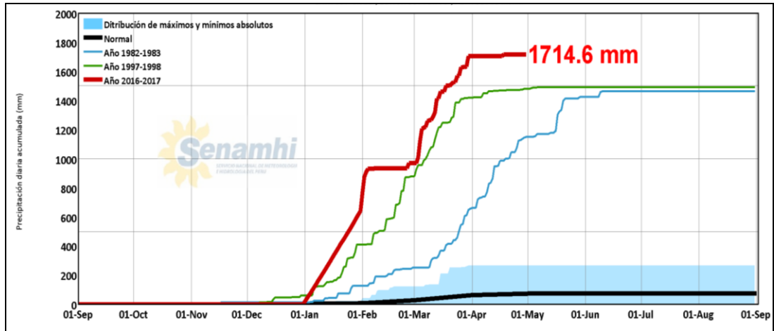
Figura 6: Precipitación diaria acumulada en la estación meteorológica Jayanca
