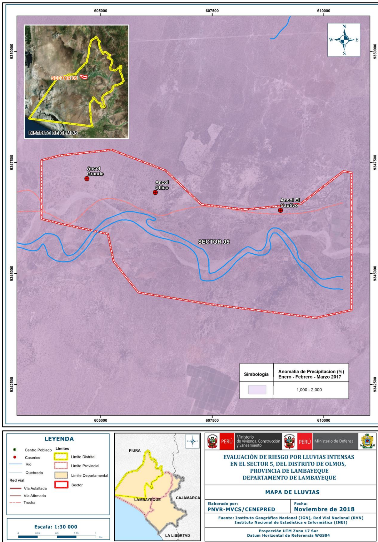
Figura 7: Anomalías de lluvias durante El Niño Costero 2017 (Enero-Marzo) para el Sector 5 del distrito Olmos.
