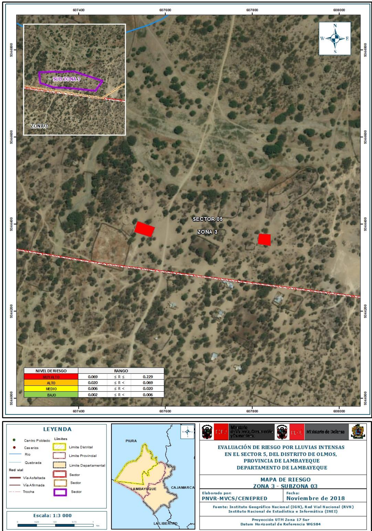
Figura 29: Mapa de Riesgo del Sector 5, distrito de Olmos – Zona 3-Sub Zona 03
