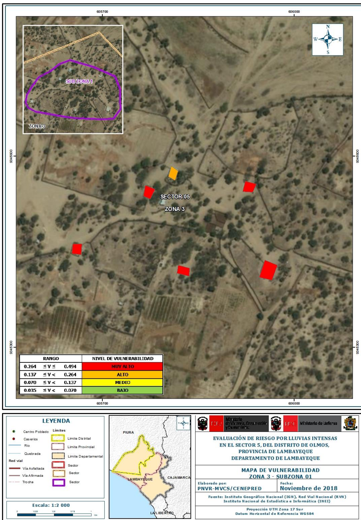
Figura 17: Mapa de Vulnerabilidad del Sector 5, distrito de Olmos – Zona 3-Sub Zona 01
