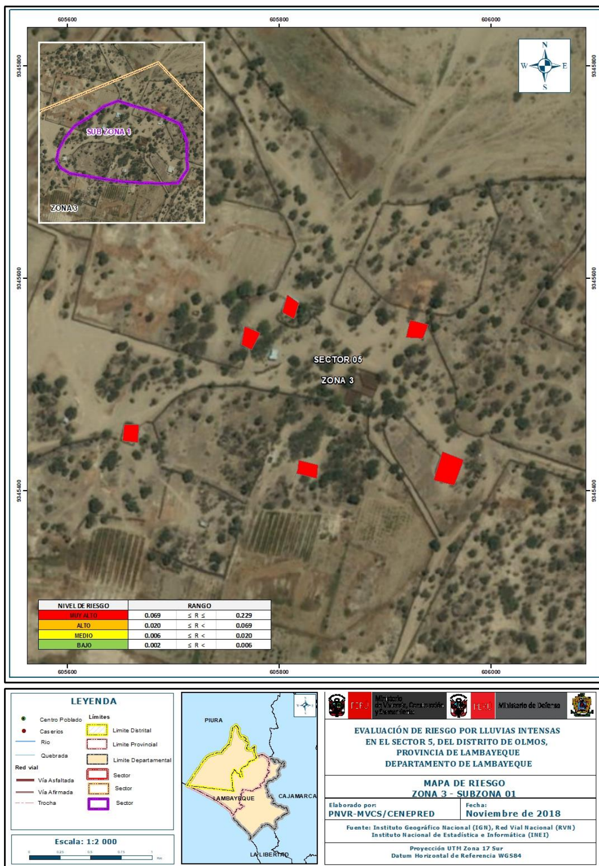
Figura 27: Mapa de Riesgo del Sector 5, distrito de Olmos – Zona 3-Sub Zona 01
