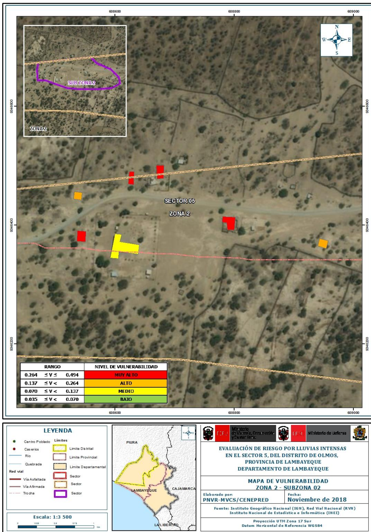
Figura 15: Mapa de Vulnerabilidad del Sector 5, distrito de Olmos – Zona 2-Sub Zona 02
