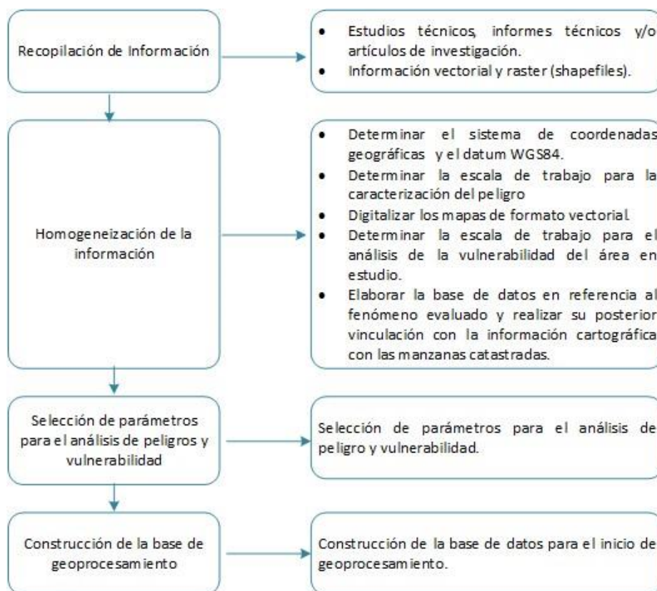
Gráfico N° 4: Flujograma general de procesos de análisis de información
