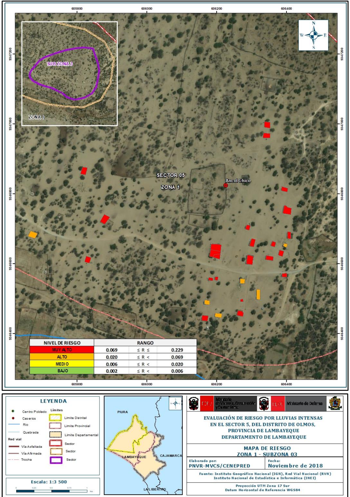
Figura 23: Mapa de Riesgo del Sector 5, distrito de Olmos – Zona 1-Sub Zona 03
