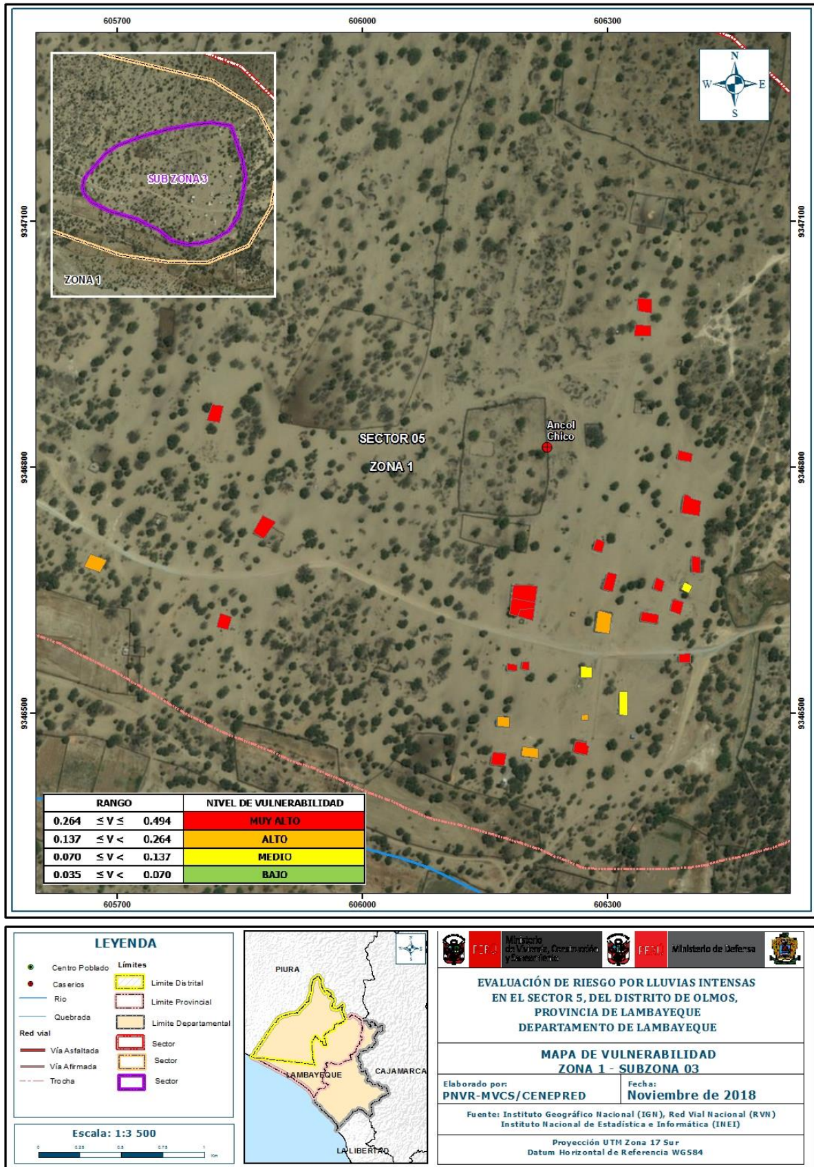
Figura 13: Mapa de Vulnerabilidad del Sector 5, distrito de Olmos –Zona 1 - Sub Zona 03
