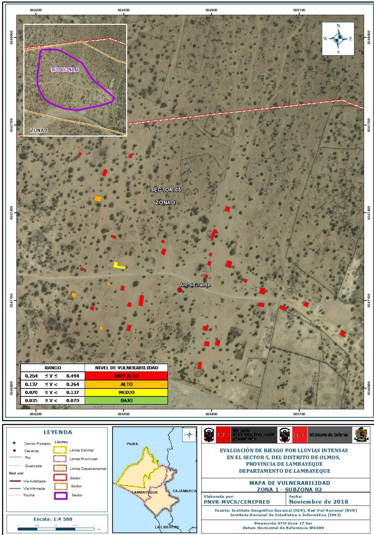
Figura 12: Mapa de Vulnerabilidad del Sector 5, distrito de Olmos – Zona 1-Sub Zona 02
