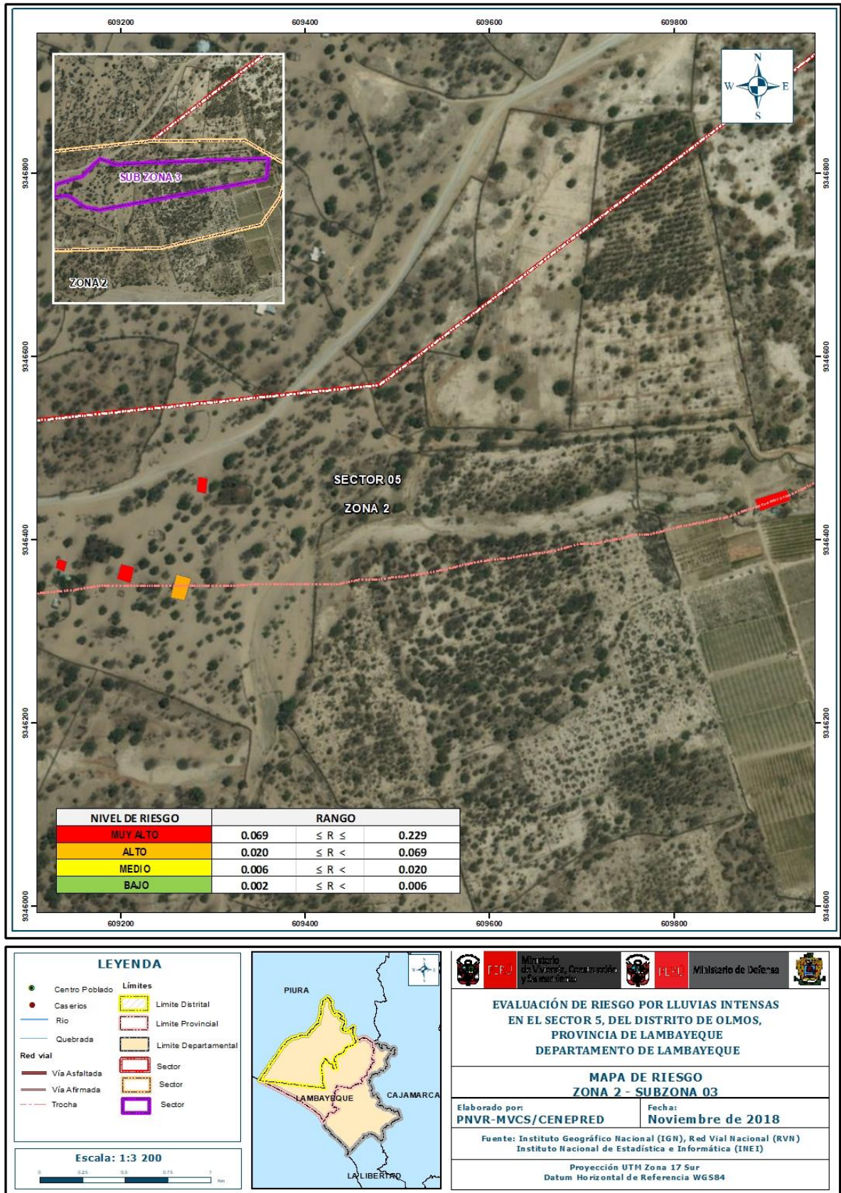
Figura 26: Mapa de Riesgo del Sector 5, distrito de Olmos – Zona 2-Sub Zona 03
