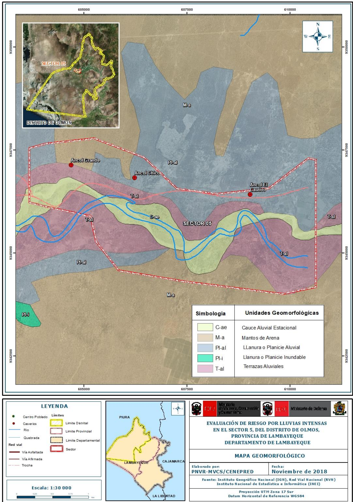
Figura 3: Mapa Geomorfológico del Sector 5
