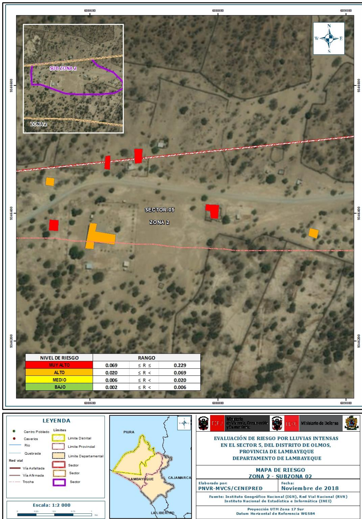
Figura 25: Mapa de Riesgo del Sector 5, distrito de Olmos – Zona 2-Sub Zona 02
