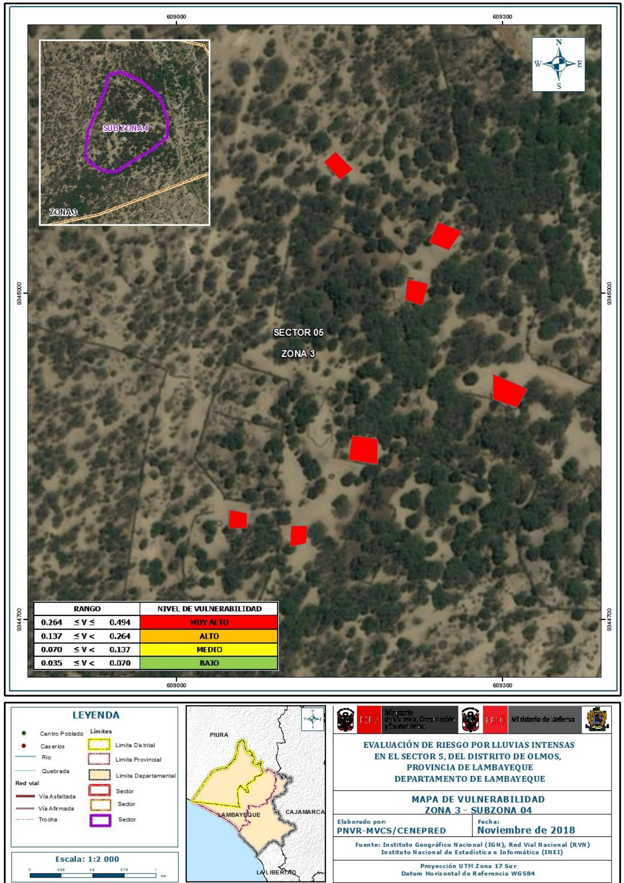
Figura 20: Mapa de Vulnerabilidad del Sector 5, distrito de Olmos – Zona 3-Sub Zona 04
