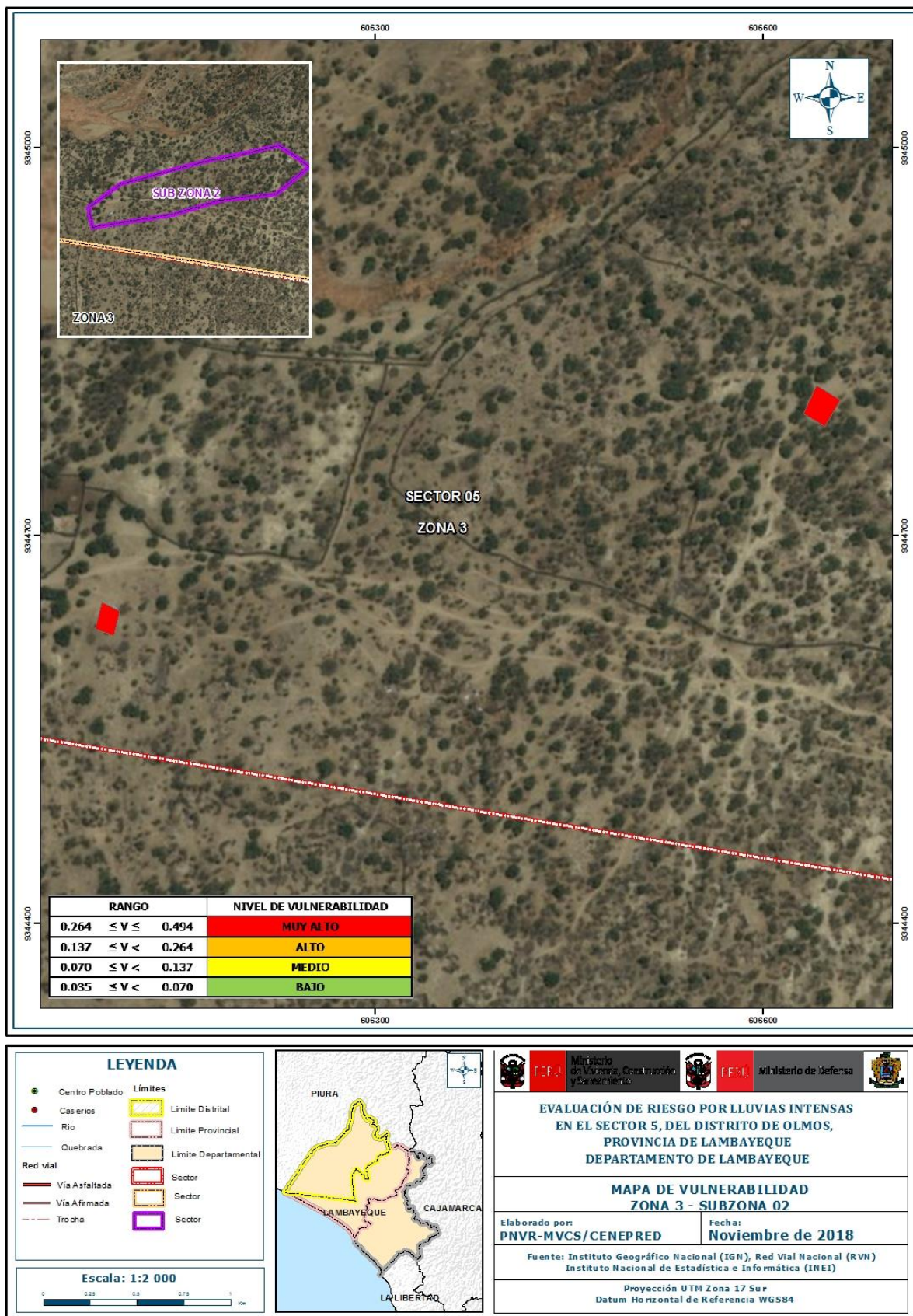
Figura 18: Mapa de Vulnerabilidad del Sector 5, distrito de Olmos – Zona 3-Sub Zona 02
