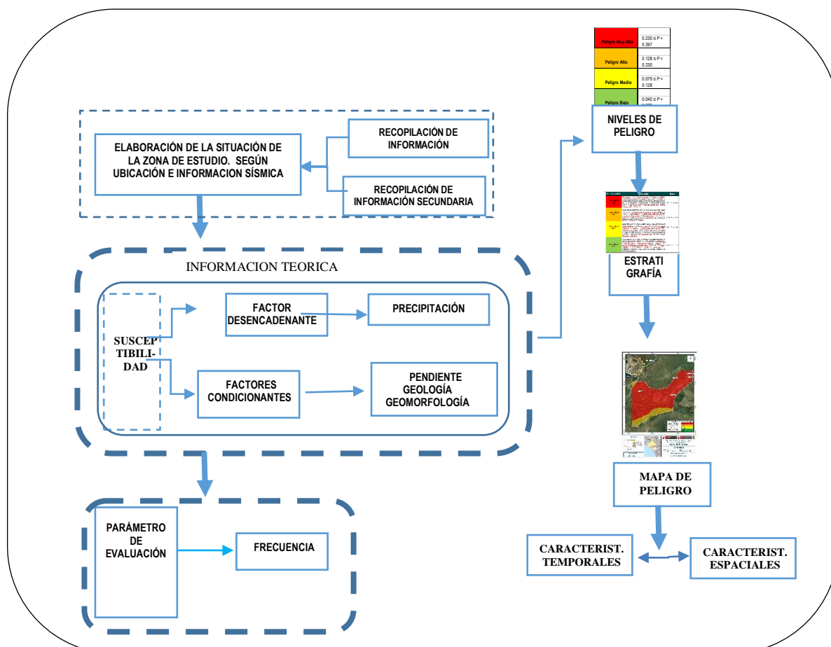
Gráfico N° 3: Metodología para la determinación de Peligrosidad
