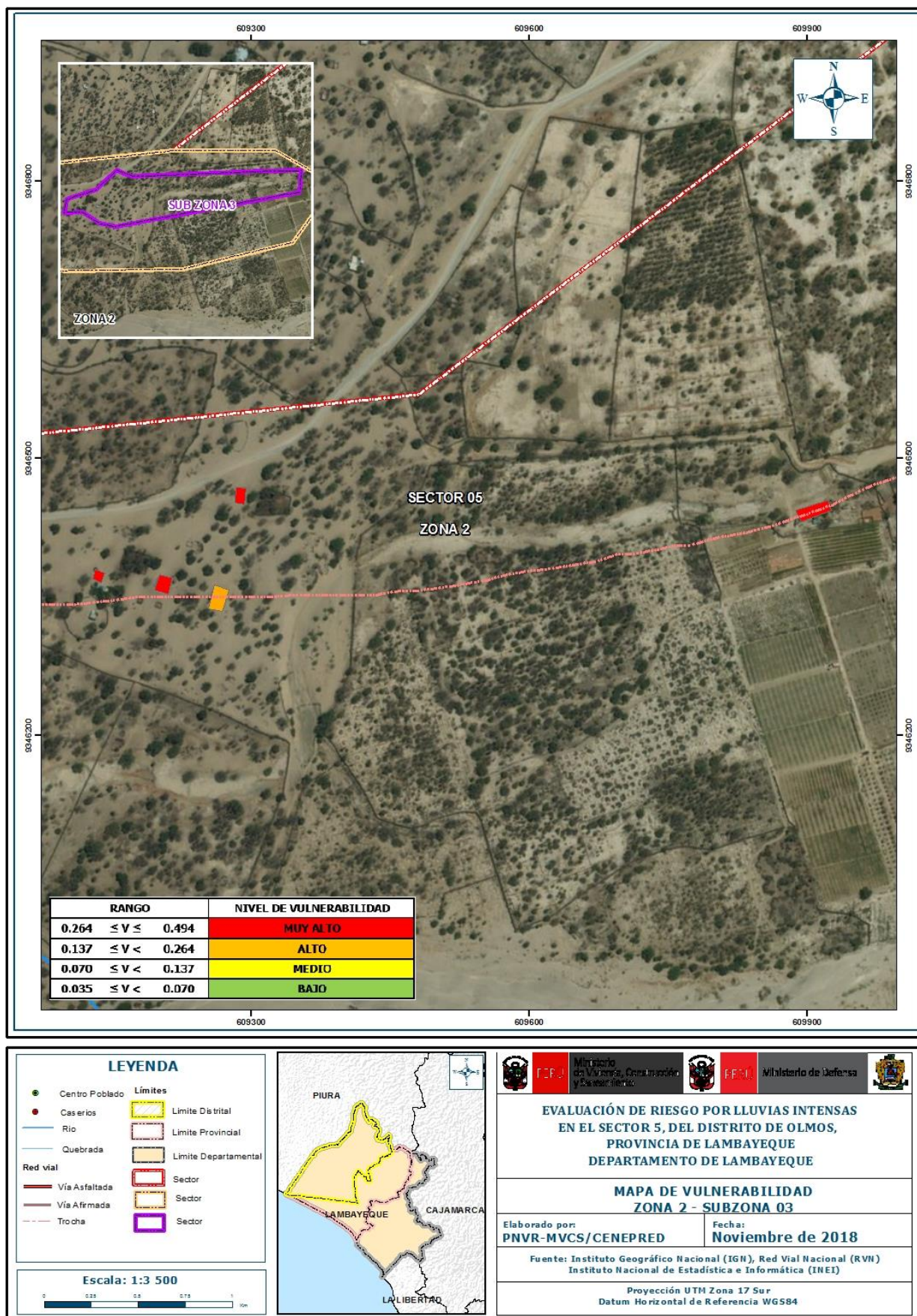
Figura 16: Mapa de Vulnerabilidad del Sector 5, distrito de Olmos – Zona 2-Sub Zona 03
