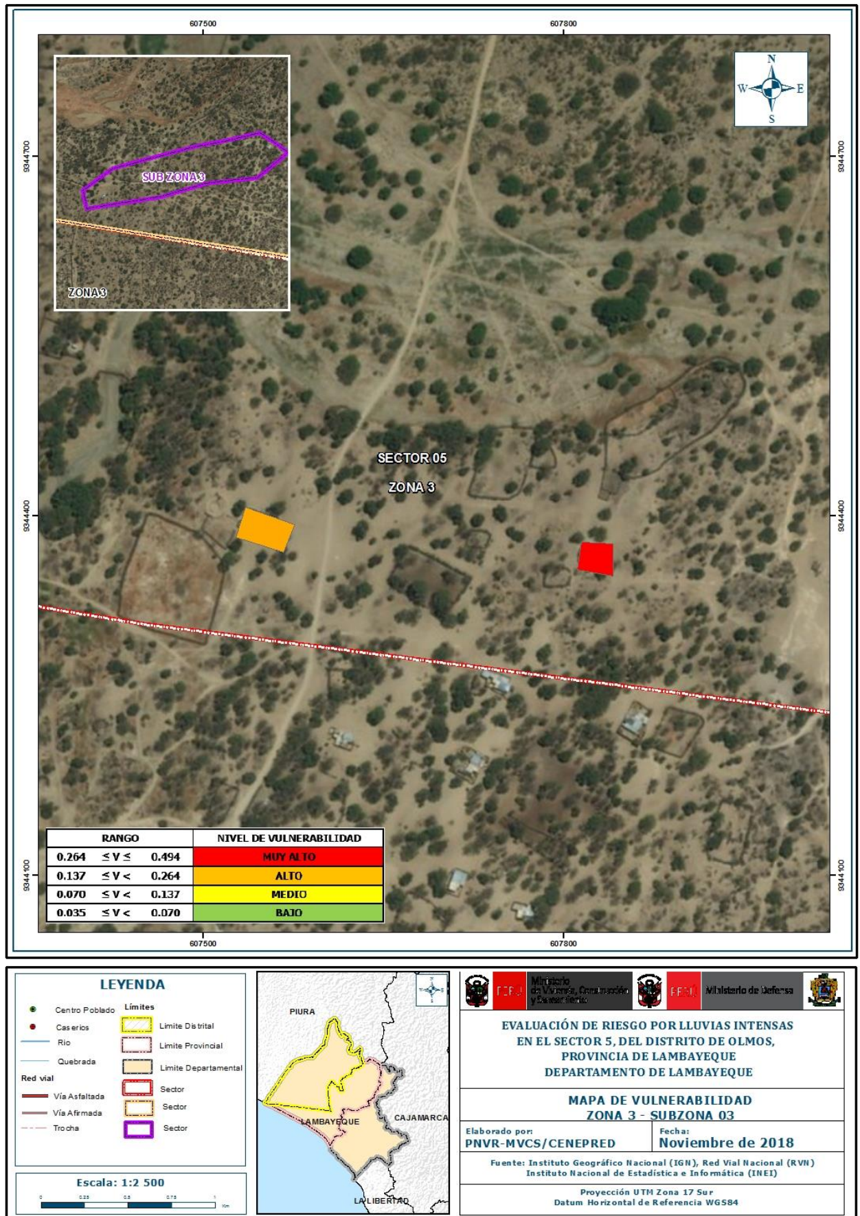
Figura 19: Mapa de Vulnerabilidad del Sector 5, distrito de Olmos – Zona 3-Sub Zona 03
