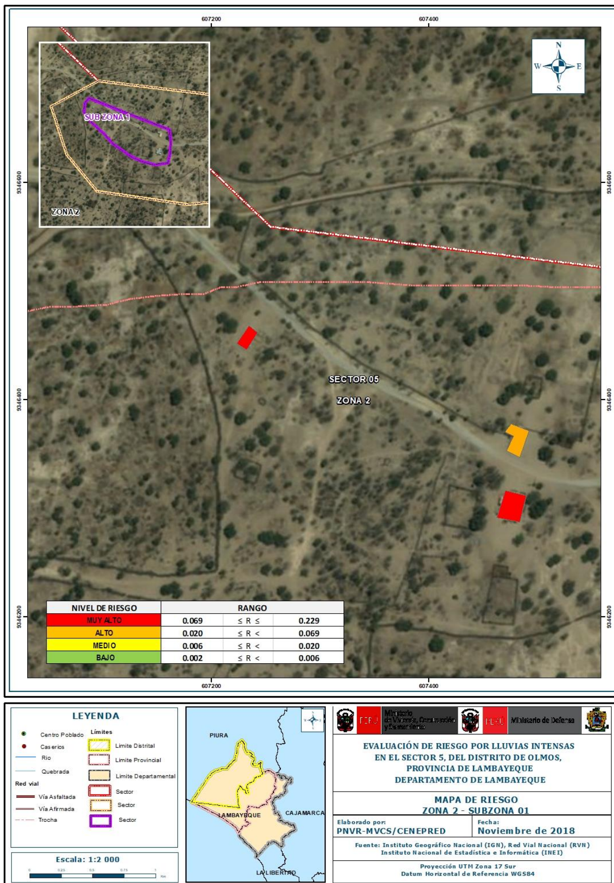
Figura 24: Mapa de Riesgo del Sector 5, distrito de Olmos – Zona 2-Sub Zona 01
