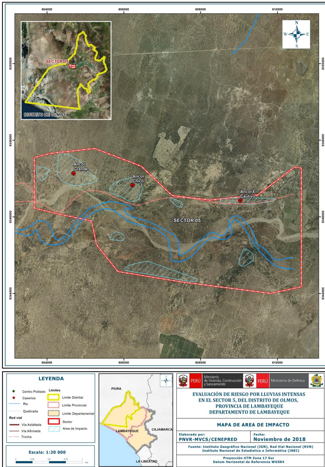
Figura 31: Mapa de Área impactada por El Niño Costero 2017 – Sector 5 del distrito de Olmos
