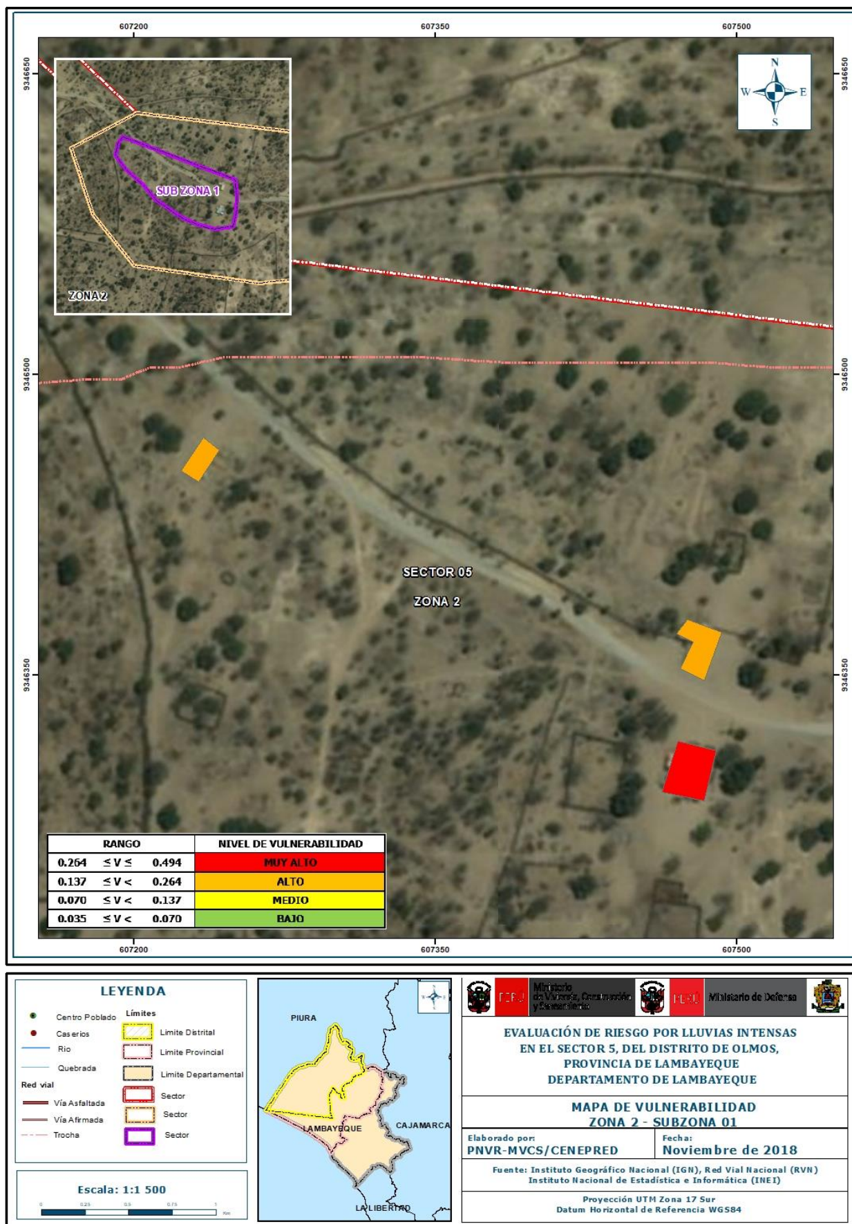
Figura 14: Mapa de Vulnerabilidad del Sector 5, distrito de Olmos – Zona 2-Sub Zona 01
