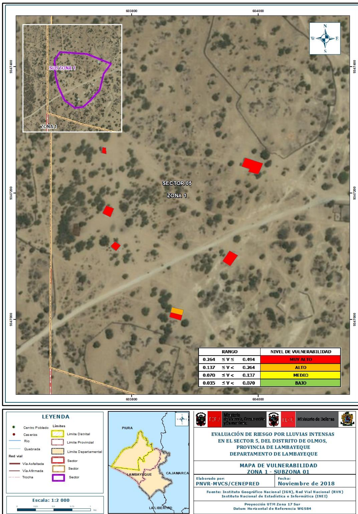
Figura 11: Mapa de Vulnerabilidad del Sector 5, distrito de Olmos – Zona 1-Sub Zona 01
