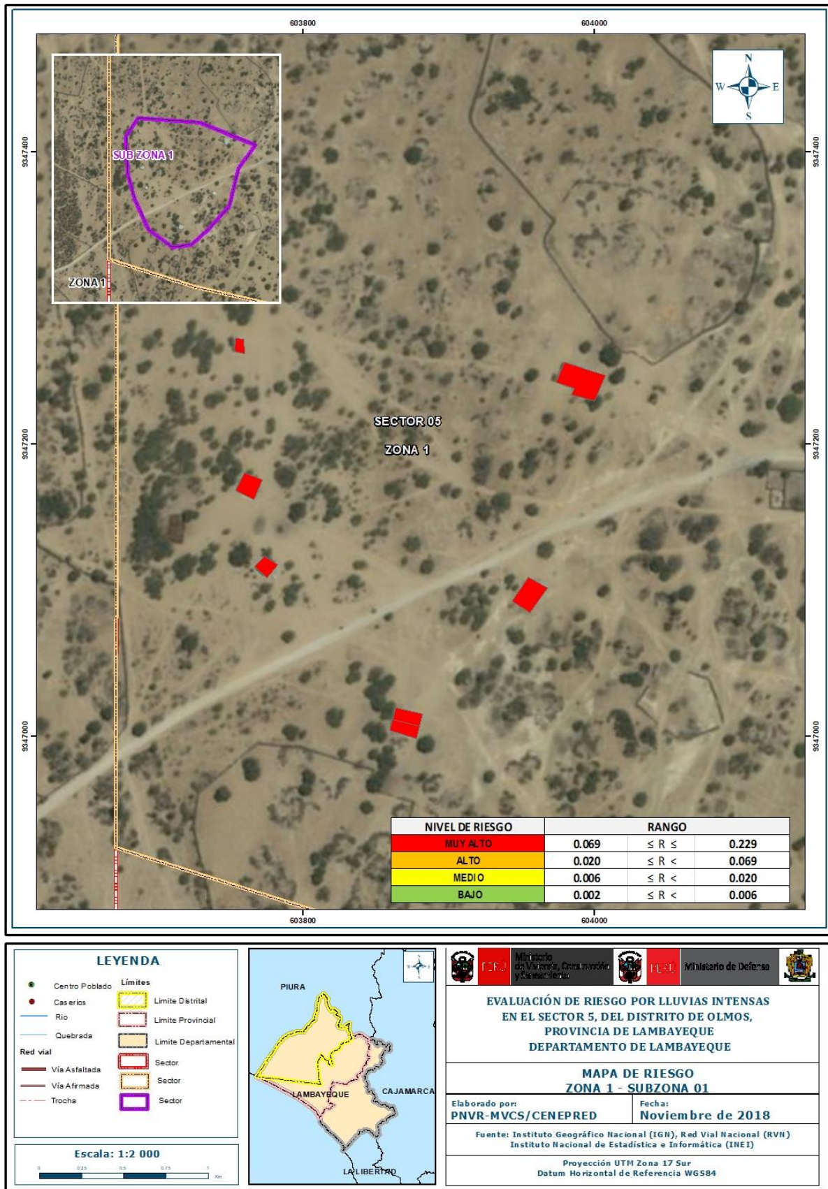
Figura 21: Mapa de Riesgo del Sector 5, distrito de Olmos – Zona 1-Sub Zona 01
