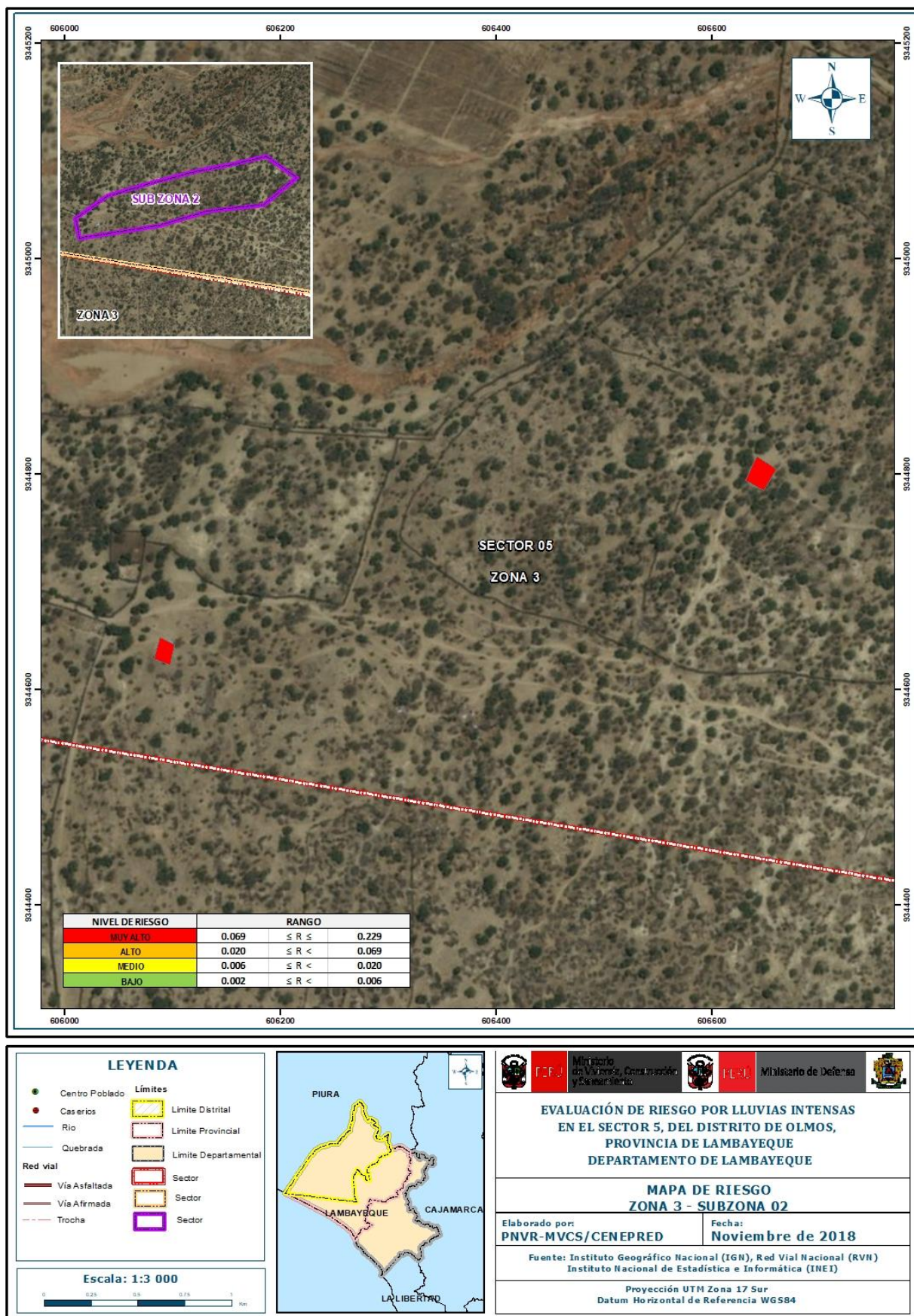
Figura 28: Mapa de Riesgo del Sector 5, distrito de Olmos – Zona 3-Sub Zona 02
