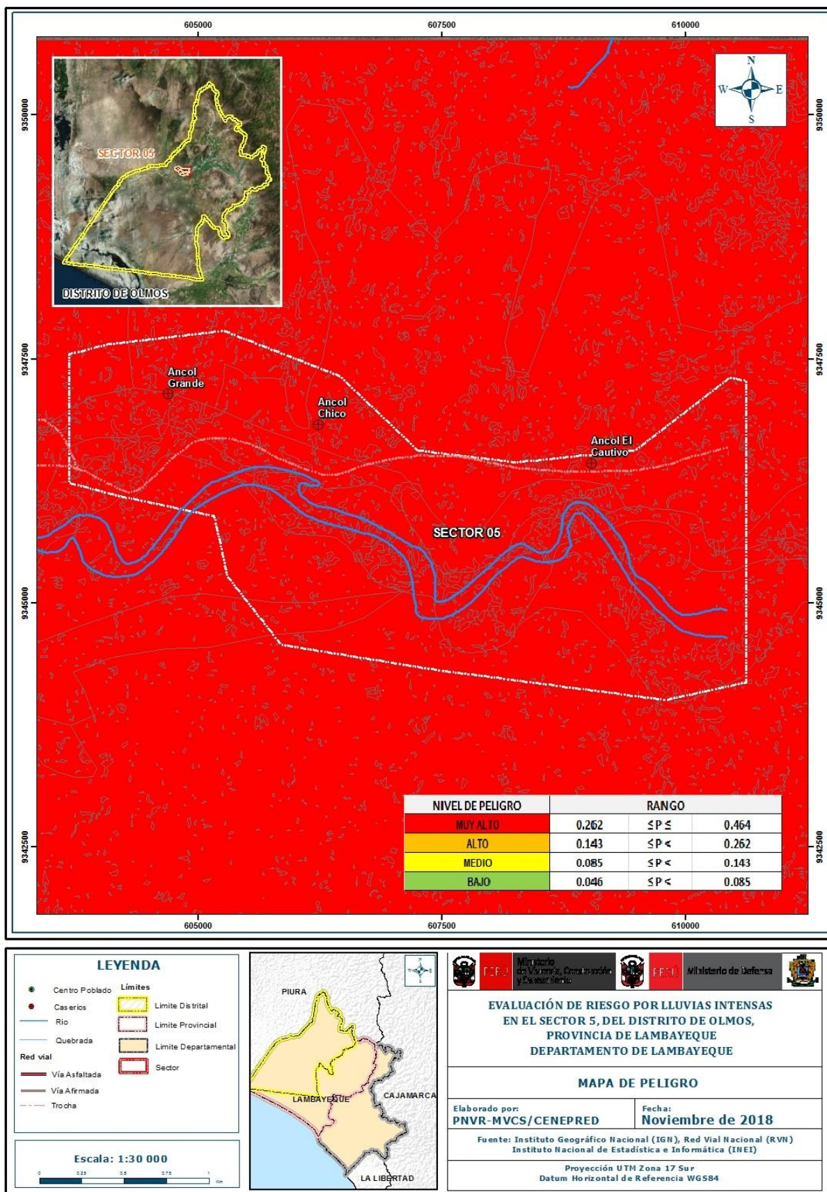
Figura 10: Mapa de Peligro del Sector 5, distrito de Olmos
