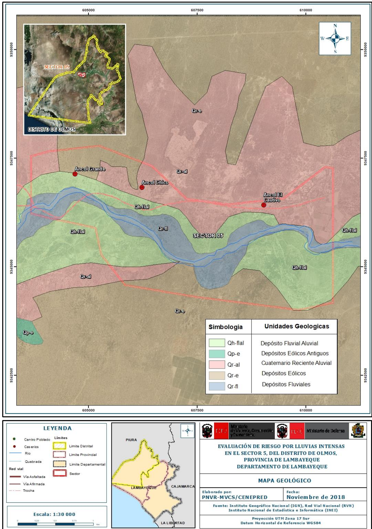
Figura 2: Mapa de Geología del Sector 5
