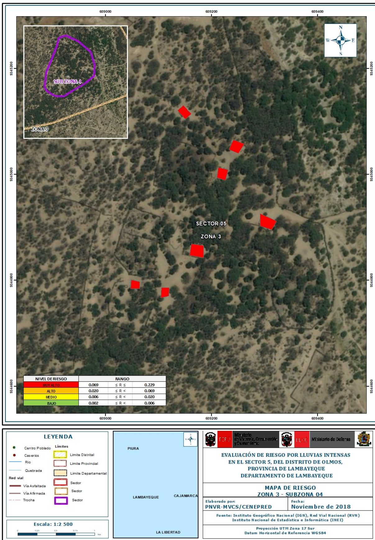
Figura 30: Mapa de Riesgo del Sector 5, distrito de Olmos – Zona 3-Sub Zona 04
