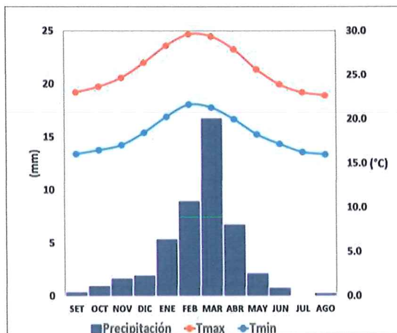
Gráfico N° 35. Comportamiento temporal de la temperatura del aire y precipitación promedio en la estación meteorológica Lambayeque
