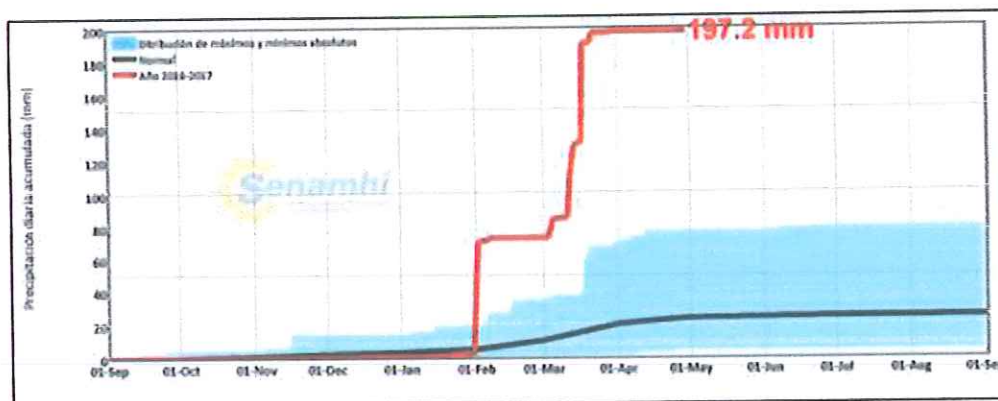
Figura N° 7. Precipitación diaria acumulada en la estación meteorológica Lambayeque
