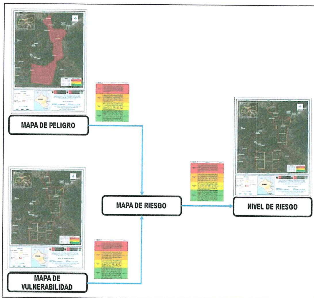
Figura N° 5: Flujograma para estimar los niveles del riesgo
