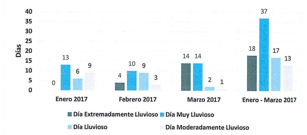
Gráfico N° 10: Frecuencia promedio de lluvias extremas durante El Niño Costero 2017 en el Sector Norte del Distrito de Pátapo
