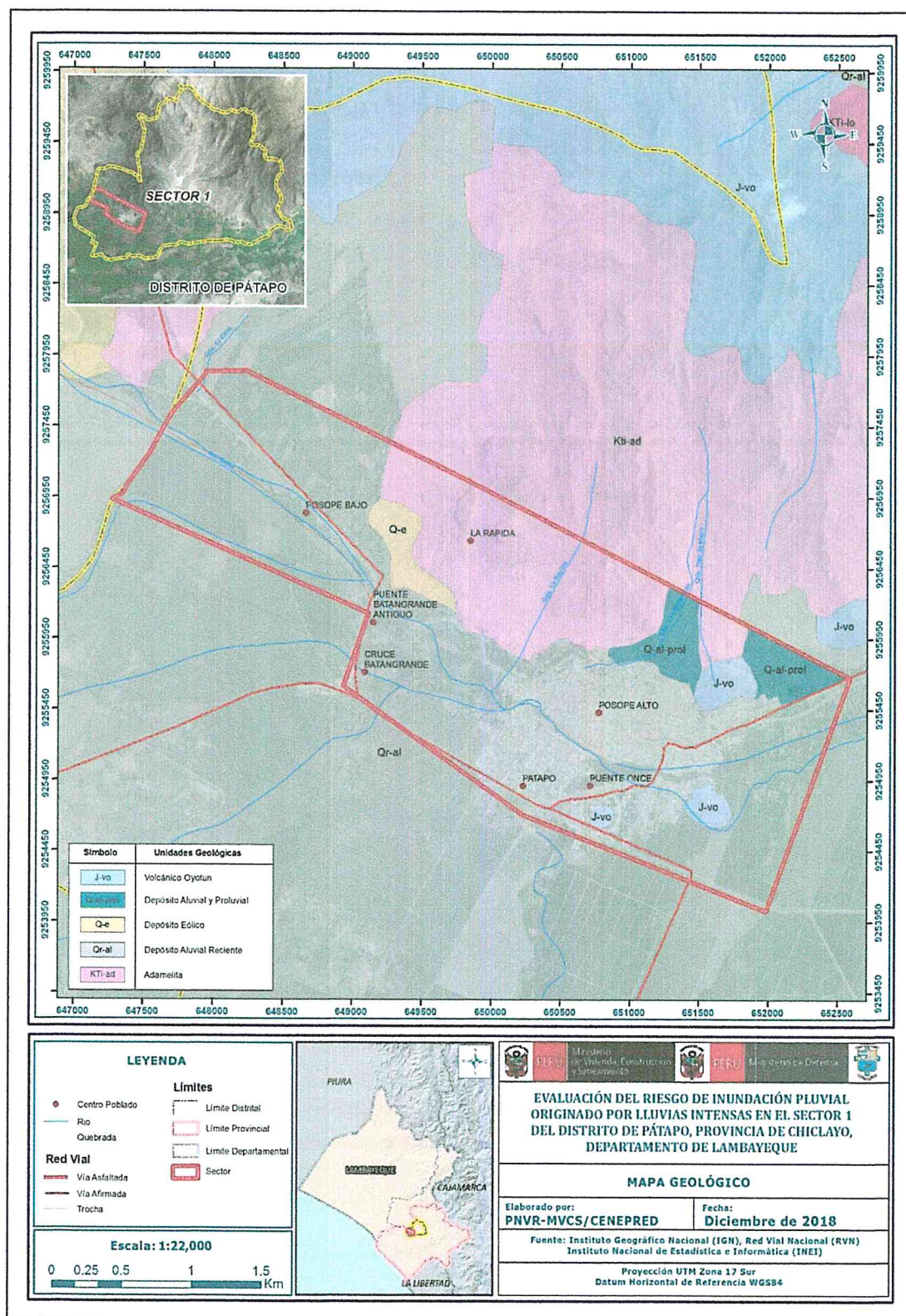
Mapa N° 2: Geológico del Sector 1 del Distrito de Pátapo
