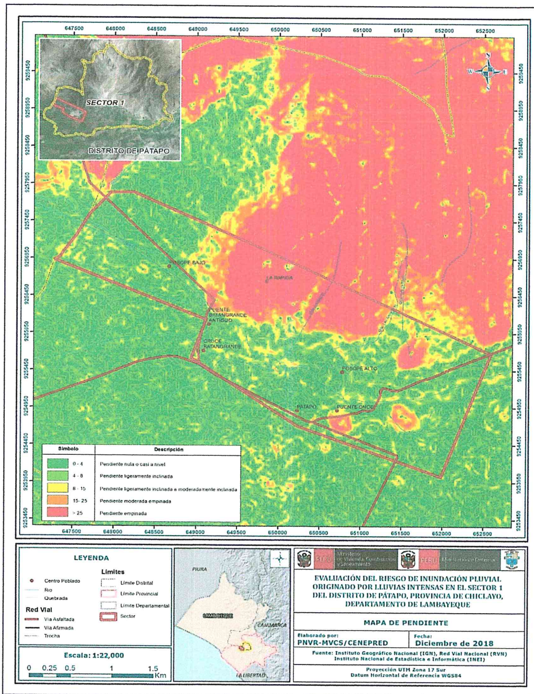
Mapa N° 4: Pendientes del sector 1 del Distrito de Pátapo
