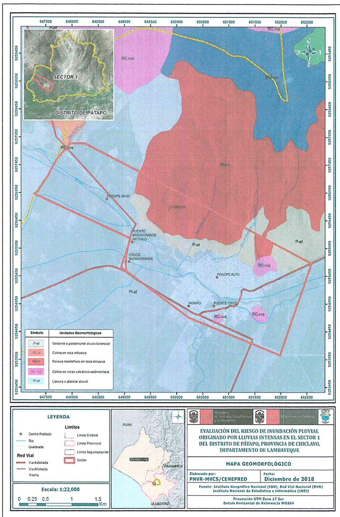
Mapa N° 3: Geomorfológico del Sector 1 del Distrito de Pátapo
