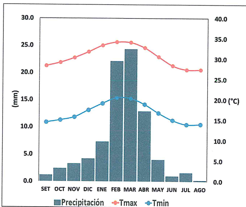
Gráfico N° 9: Comportamiento temporal de la temperatura del aire y precipitación promedio en la estación meteorológica Jayanca
