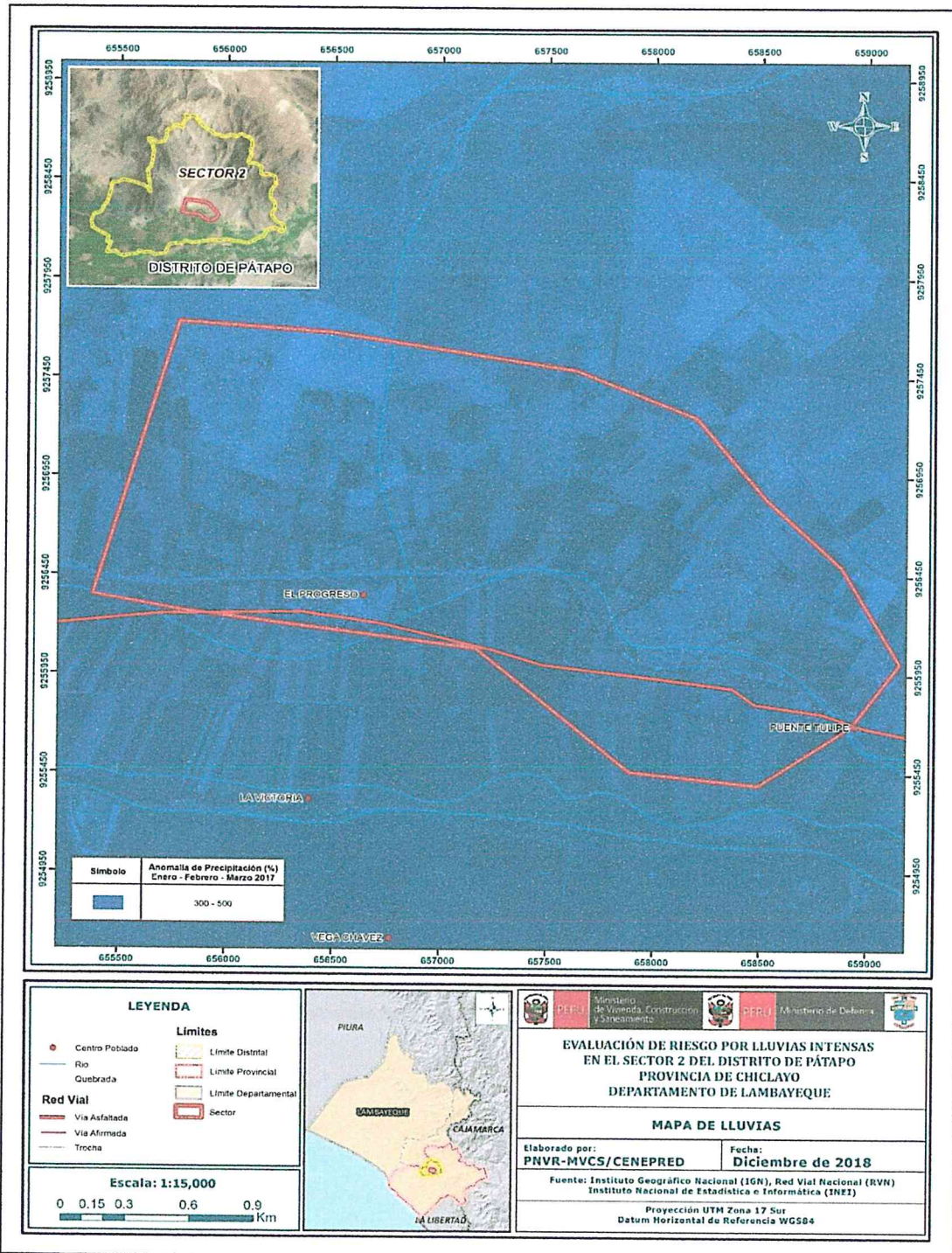
Mapa N° 5: Anomalías de lluvias durante El Niño Costero 2017 (Enero-Marzo) para el Sector 2 del distrito Pátapo.
