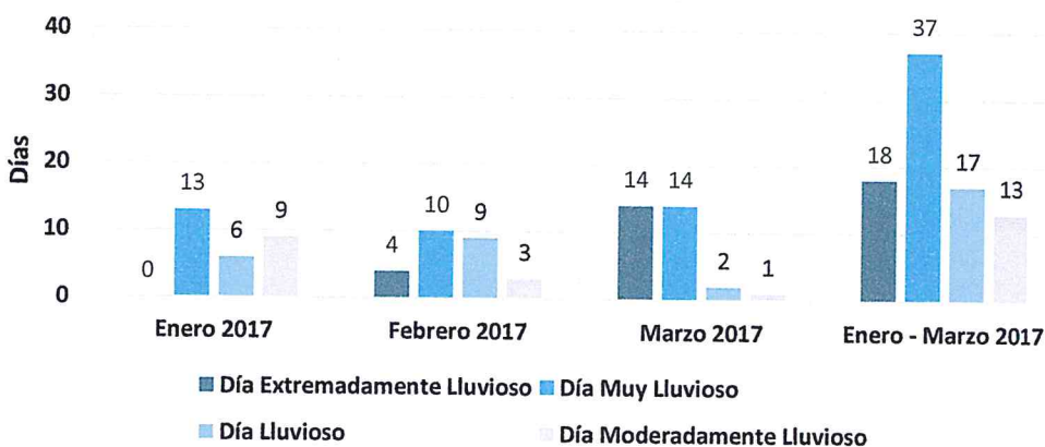
Gráfico N° 10: Frecuencia promedio de lluvias extremas durante El Niño Costero 2017 en el Sector Norte del Distrito de Pátapo
