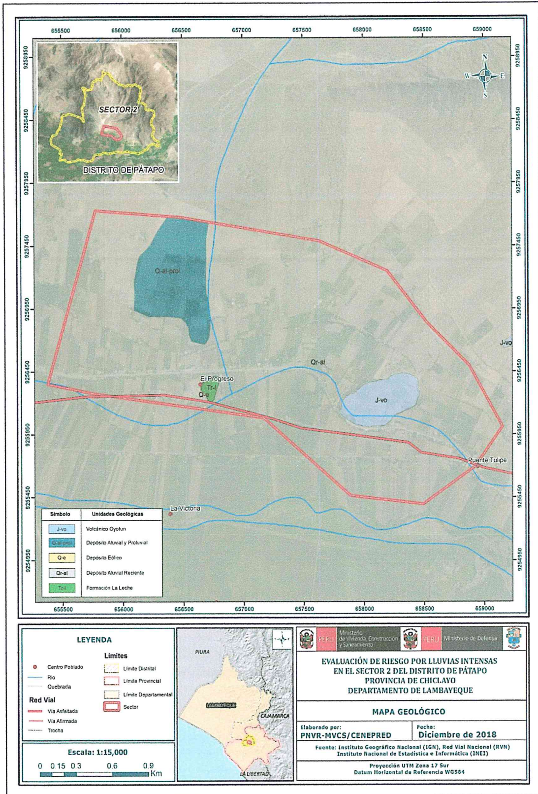
Mapa N° 2: Geológico del Sector 2 del Distrito de Pátapo
