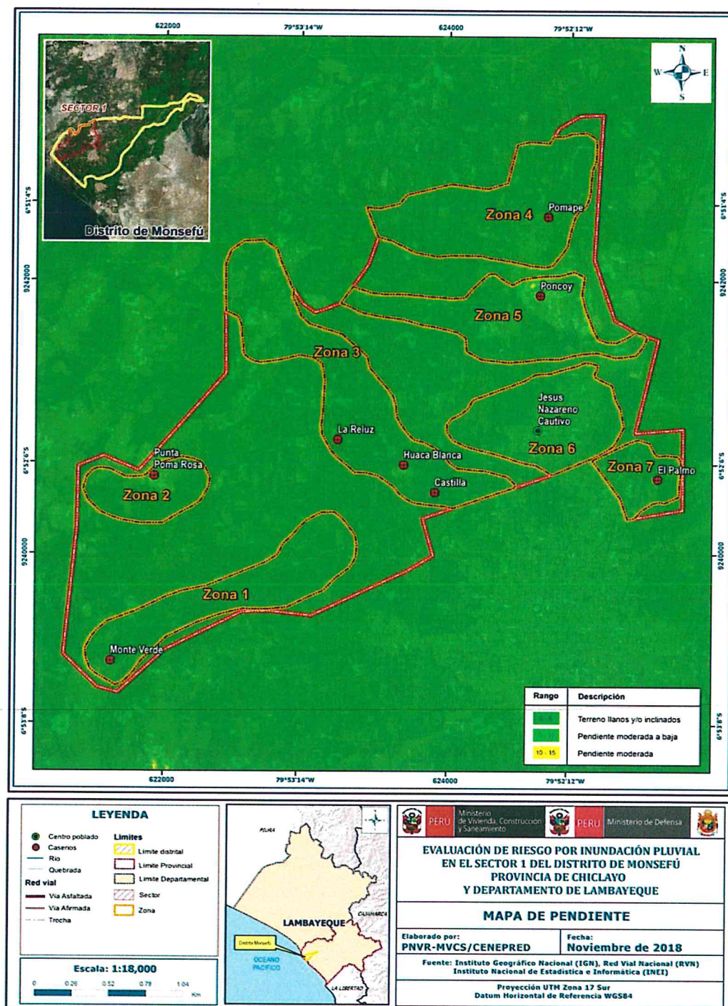
Figura 10. Mapa de Pendientes - Sector 1 - Distrito Monsefu
