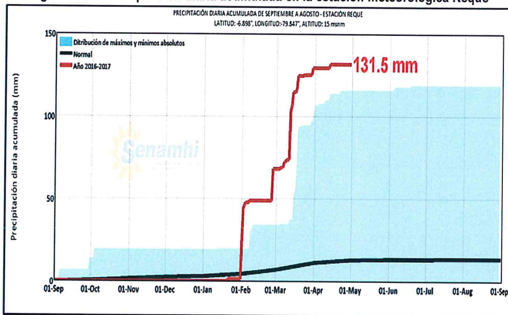
Figura N° 13. Precipitación diaria acumulada en la estación meteorológica Reque
