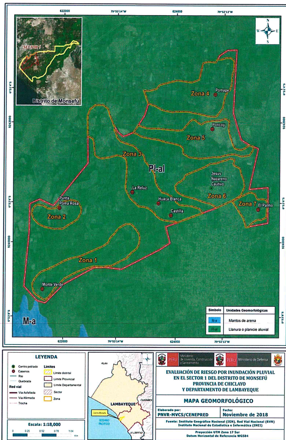
Figura 9. Mapa Geomorfológico - Sector 1- Distrito Monsefu
