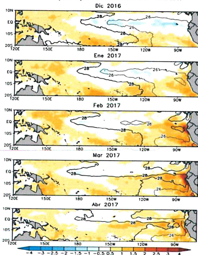
Figura N° 12. Anomalía de la Temperatura superficial del mar (°C) en el Pacífico ecuatorial para el periodo diciembre 2016 – abril 2017
