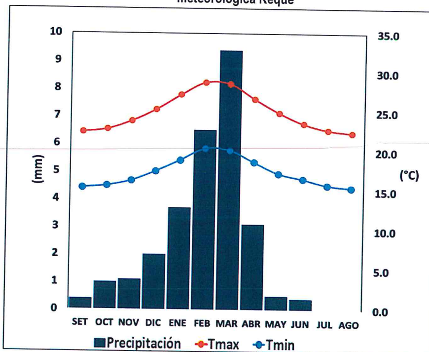
Gráfico N° 09. Comportamiento temporal de la precipitación promedio en la estación meteorológica Reque
