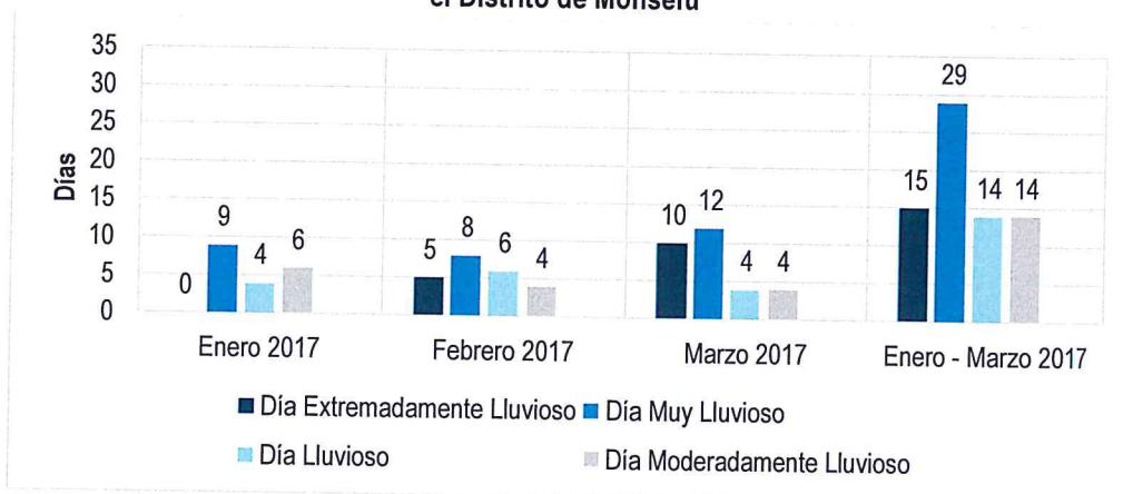
Gráfico N° 10. Frecuencia promedio de lluvias extremas durante El Niño Costero 2017 en el Distrito de Monsefú
