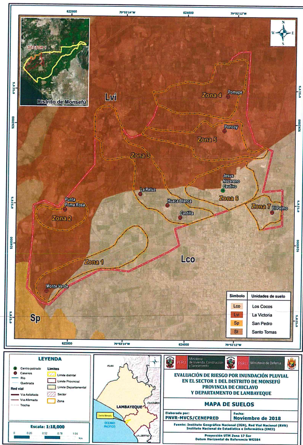
Figura 11. Mapa de Suelos - Sector 1 - Distrito Monsefú
