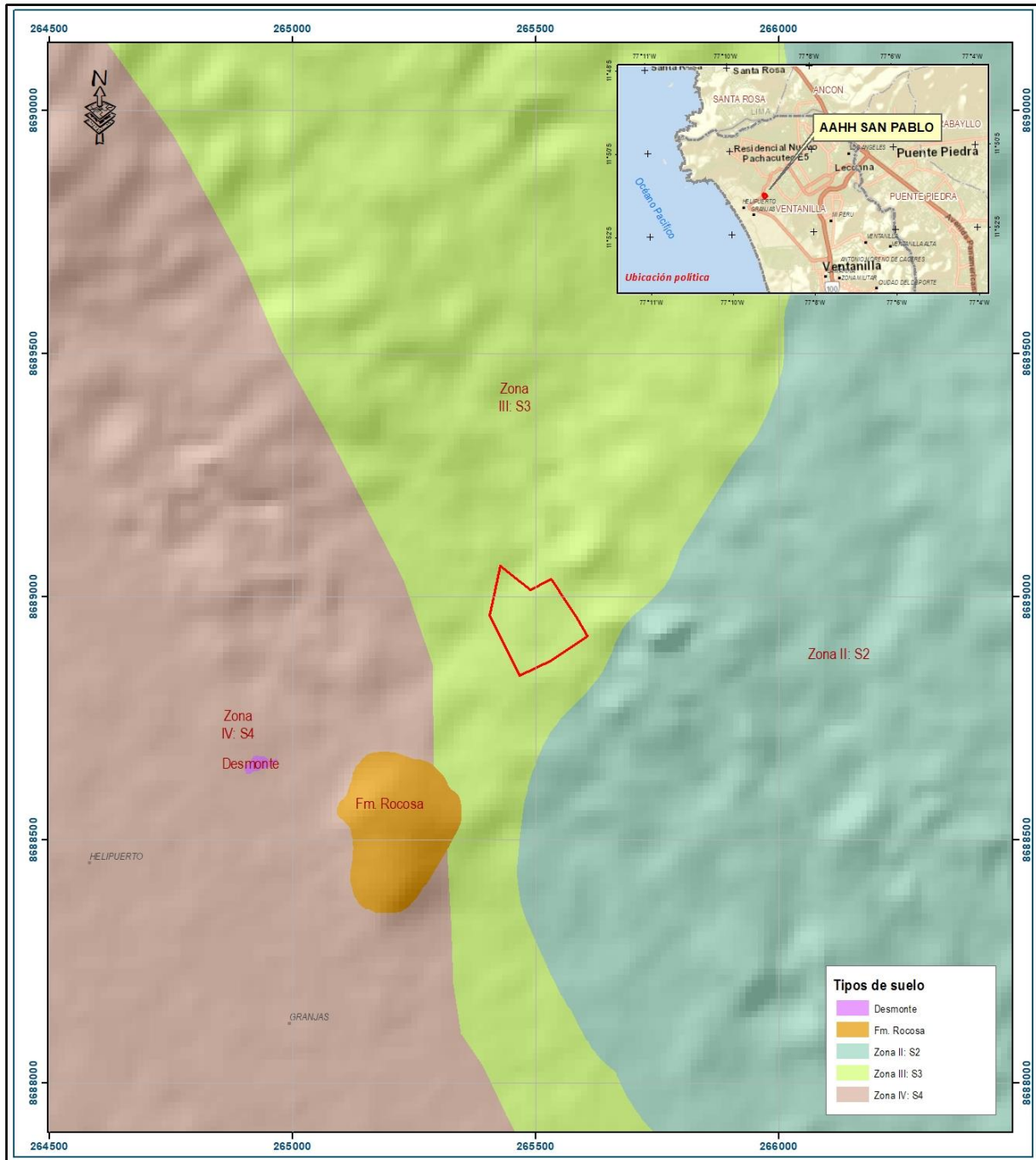
Figura N° 6. Mapa geológico del área de estudio.
