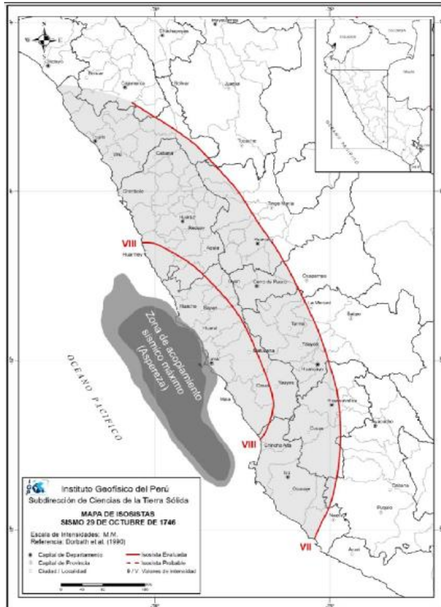
Figura N° 9: Mapa de isosistas del sismo de 1746 según Dorbath et al (1990).
