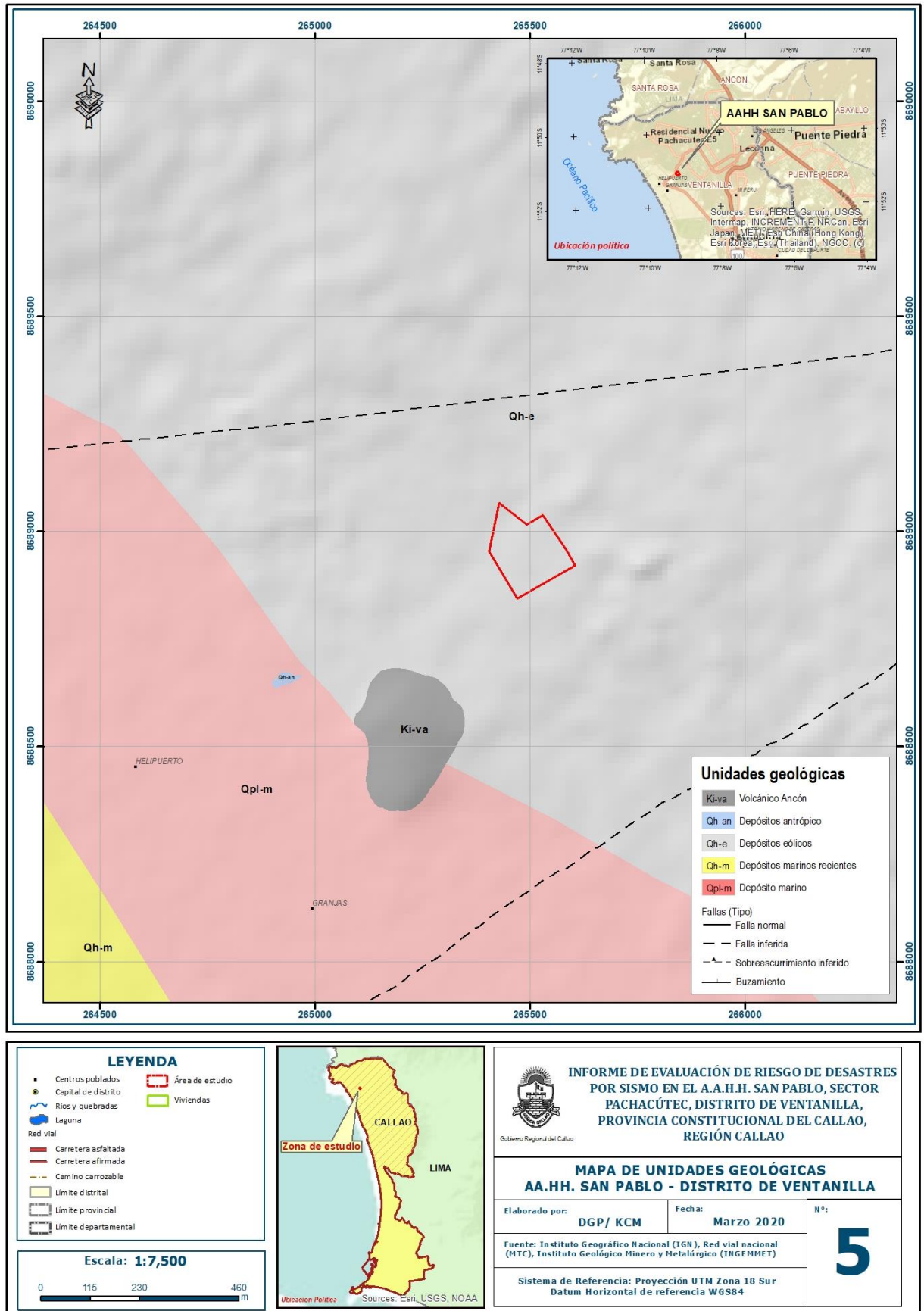
Figura N° 5. Mapa geológico del área de estudio.
