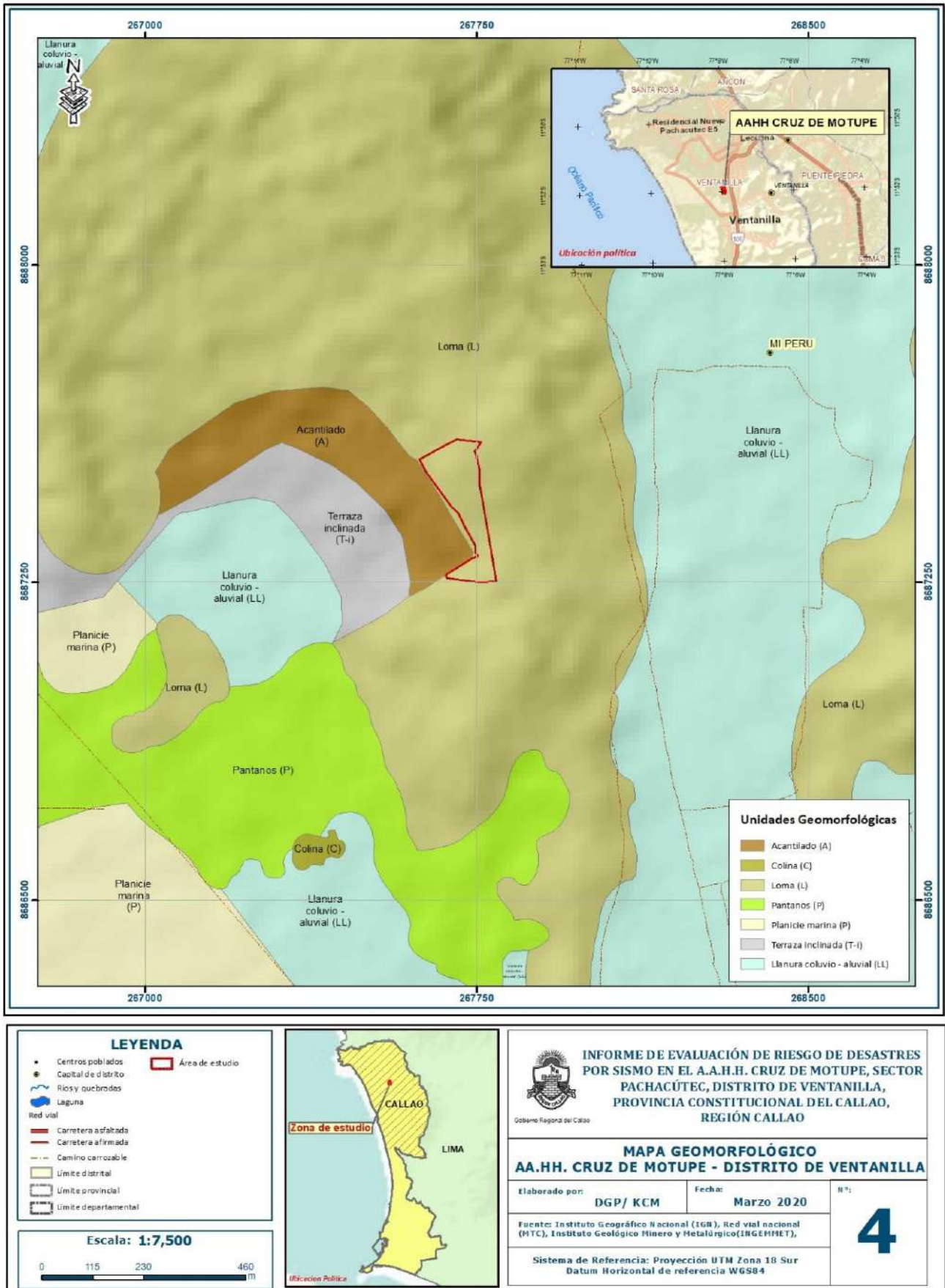
Figura N° 4. Mapa geomorfológico del área de estudio.
