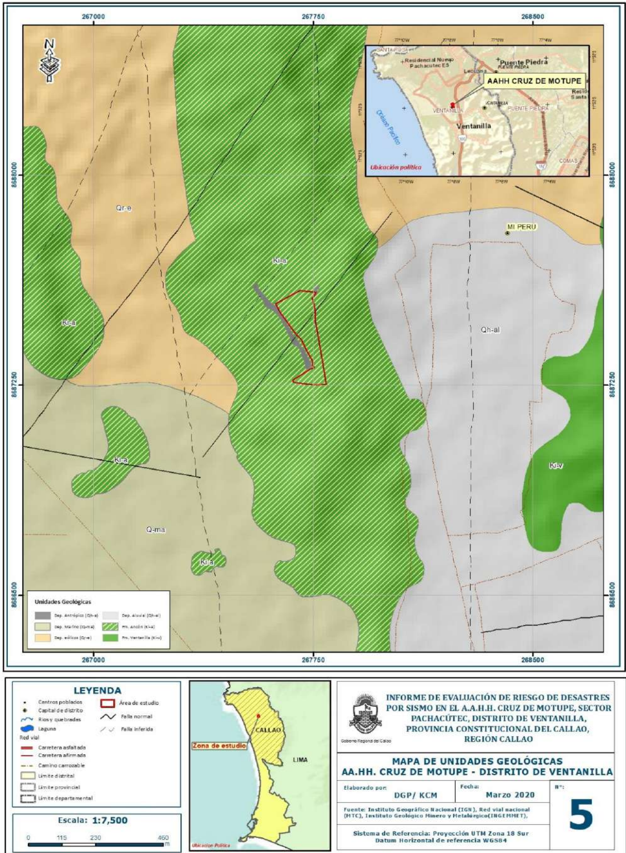
Figura N° 5. Mapa geológico del área de estudio.
