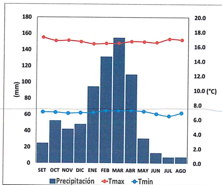
Gráfico N° 08. Comportamiento temporal de la precipitación promedio en la estación meteorológica Salpo
