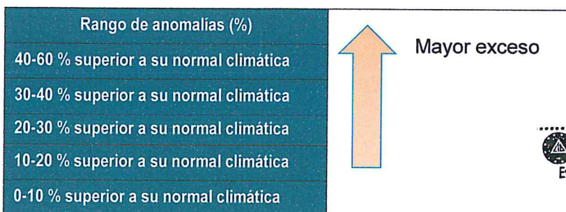
Cuadro N° 1. Anomalías de lluvia durante el periodo enero-marzo 2017 para el sector 1 del distrito Huaso
