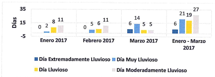
Gráfico N° 11. Frecuencia promedio de lluvias extremas durante El Niño Costero 2017 en el distrito de Huaso
