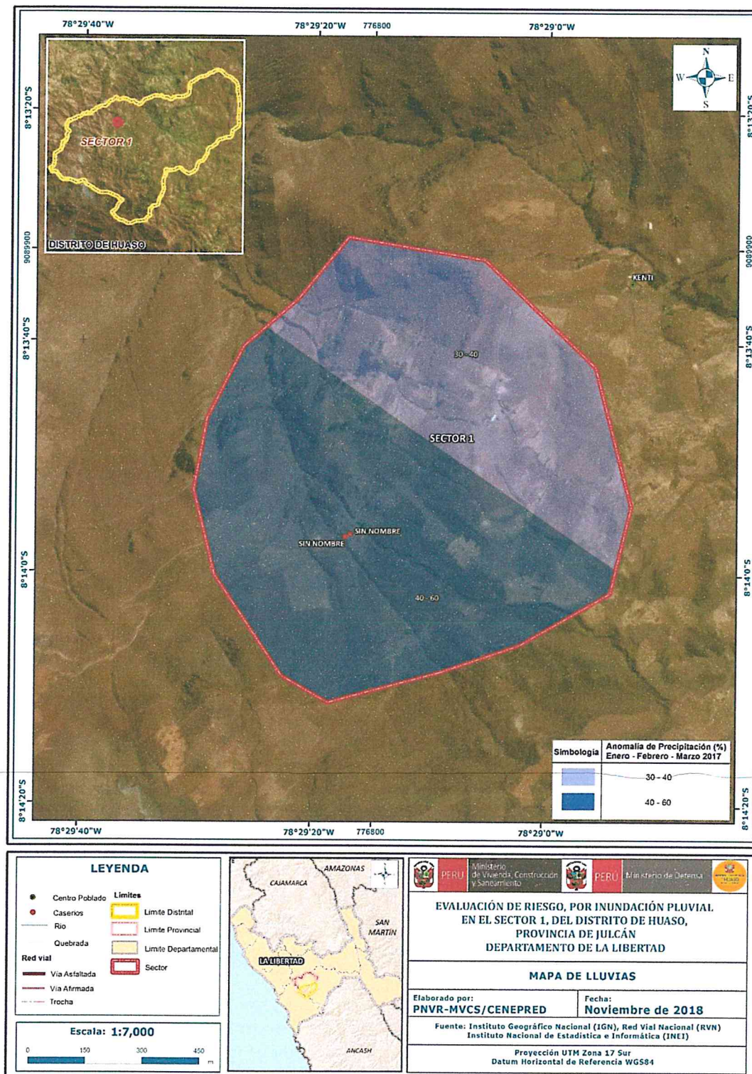
Figura N° 05 – Mapa de Anomalías de Lluvias durante El Niño Costero 2017 (Enero-Marzo) para el sector 1 del distrito Huaso
